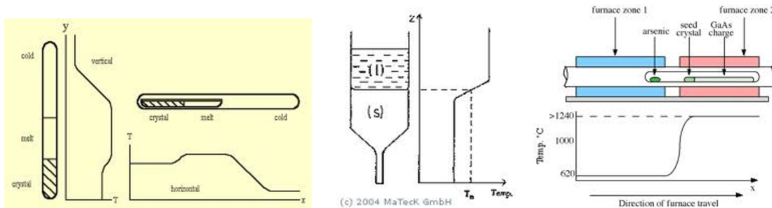
Obr.8. Bridgmanova metoda
