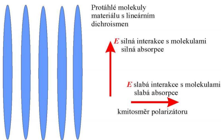
Obr. 2.9 Schématické znázornění principu dichroického polarizátoru
