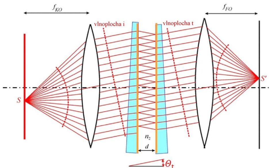
Obr. 4.21 Fabryův-Pérotův interferometr se vstupující jednou rovinnou vlnou. Intenzita obrazu S' bodového zdroje S je modulována funkcí danou vztahem (4.38). O tom, zda bude obraz intenzivní nebo naopak temný, rozhoduje při pevném nastavení d, n_2 úhel \theta_t , tedy poloha bodu S . Interferometr lze ladit právě mechanickou změnou d (např. piezoelektricky) nebo indexu lomu n_2 (např. tlakem plynu v prostoru mezi deskami). Vzhledem k osové symetrii jsou při „rozsvícení“ mnoha bodů ve fokální rovině kolimátoru pozorovány kroužky stejného sklonu. Poloha intenzitních maxim je podobná jako u jiných interferometrů, ale velmi podstatný rozdíl je v jejich vysoké ostrosti pro kvazimonochromatické záření s velmi úzkou spektrální čarou.
