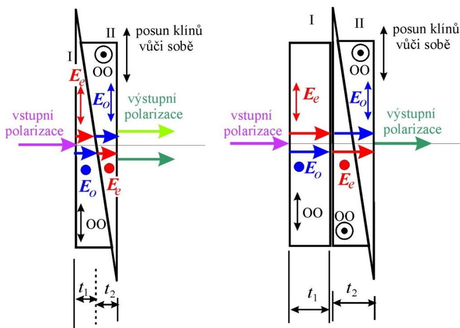
Obr. 10.12 Babinetův a Babinetův-Soleilův kompenzátor s vyznačenými směry optických os dvojlomného materiálu a kmity elektrického pole. Červeně je vyznačena mimořádná vlna (index lomu n_e ) a modře vlna řádná (index lomu n_o ) v daných částech kompenzátoru. OO značí směr optické osy. Mechanickým posunem klínů se mění délka optické dráhy, kterou světlo proběhne částmi kompenzátoru. Tím se mění fázový posun obou složek polarizace. Jedná se o fázovou destičku s proměnnou tloušťkou. V Babinetově kompenzátoru je v ploše různý rozdíl tloušťek klínů a proto z různých míst vystupuje poněkud odlišná polarizace.
