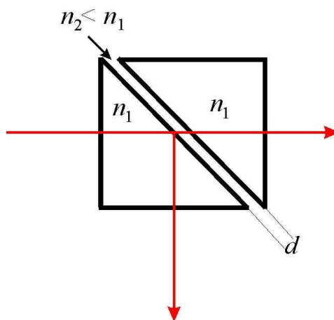
Obr. 3.13 Dvojhranol s mezerou, který může pracovat jako dělič svazku nebo jako regulovatelný vazební člen. Poměr mezi intenzitami vystupujících svazků lze regulovat šířkou štěrbinu d .
