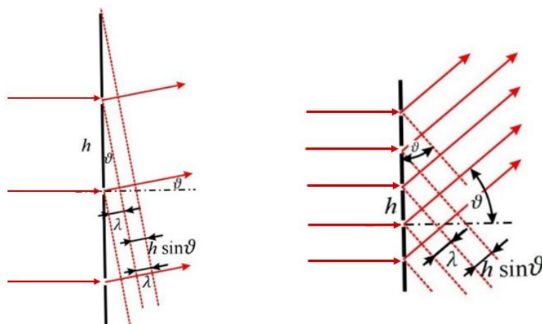
Obr 6.25 Souvislost mezi úhlem \vartheta_{MAX\ 1} a vzdáleností štěrbin. Pro velká h je dosaženo podmínky maxima h \sin \vartheta_{MAX\ 1} = \lambda pro m = 1 při menších úhlech \vartheta než pro malá h .
