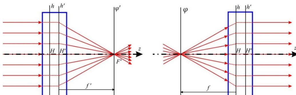
Obr. 8.13 Hlavní body H, H' a ohniska F, F' ideální dioptrické soustavy v paraxiální aproximaci. Obrázek je nakreslen pro stejné indexy lomu na obou stranách soustavy, kdy platí f' = -f . Kvůli přehlednosti obrázku nesplňují zakreslené paprsky paraxiální podmínku.
