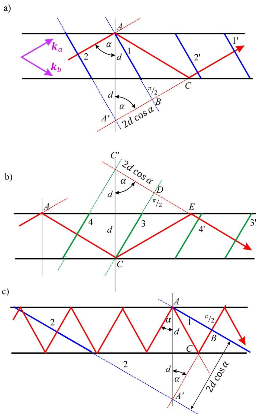
Obr. 9.3 a) Geometrická konstrukce k určení dráhového rozdílu mezi vlnoplochy procházejícími body A a A'. Paprsky jsou kresleny červeně a vlnoplochy modře. Vlnoplochy 1 a 2 jsou zakresleny pro jeden okamžik, vlnoplochy 1' a 2' znázorňují jejich polohu v pozdějším čase. Trojúhelník ABA' je pravoúhlý s přeponou AA' délky 2d a odvěsna A'B má délku 2d \cos \alpha . Nakresleno pro případ velkého úhlu \alpha a paprsky směřující k horní části obrázku. b) Určení dráhového rozdílu mezi vlnoplochy procházejícími body C a C'. Paprsky jsou kresleny červeně a vlnoplochy zeleně. Pro případ velkého úhlu \alpha a paprsky směřující k dolní části obrázku. c) Pro malý úhel \alpha , který ovšem ještě musí splňovat podmínku totálního odrazu. V obrázku a) jsou zakresleny i vlnové vektory interferujících rovinných vln: \mathbf{k}_a se vztahuje k modrým vlnoplochám na obr. a) a \mathbf{k}_b se vztahuje k zeleným vlnoplochám na obr. b).
