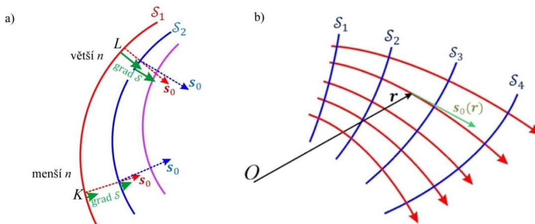
Obr. 8.4 a) Znáznornění řezů plochami eikonálů o hodnotách \mathcal{S}_1 (červeně) a \mathcal{S}_2 (modře). Zeleně jsou zakresleny gradienty eikonálu v místech K a L. V místě K jsou \mathcal{S}_1 a \mathcal{S}_2 od sebe vzdálenější než v místě L, takže gradient je v K menší než v L. To je přímo určeno indexem lomu n , který je v oblasti K menší než v oblasti L. Vlnoplochy v místě K běží rychleji než v místě L. Směry paprsků \mathbf{s}_0 jsou rovnoběžné s \text{grad } \mathcal{S} ; v obrázku jsou z důvodu přehlednosti poněkud posunuty. Směry paprsků jsou stáčeny do oblasti prostoru s větším indexem lomu. b) Řezy plochami konstantních eikonálů (modře) a paprsky (červeně) pro jiné prostorové rozložení indexu lomu než v obr. a). Tečna \mathbf{s}_0(\mathbf{r}) k paprsku v místě \mathbf{r} je naznačena zeleně.
