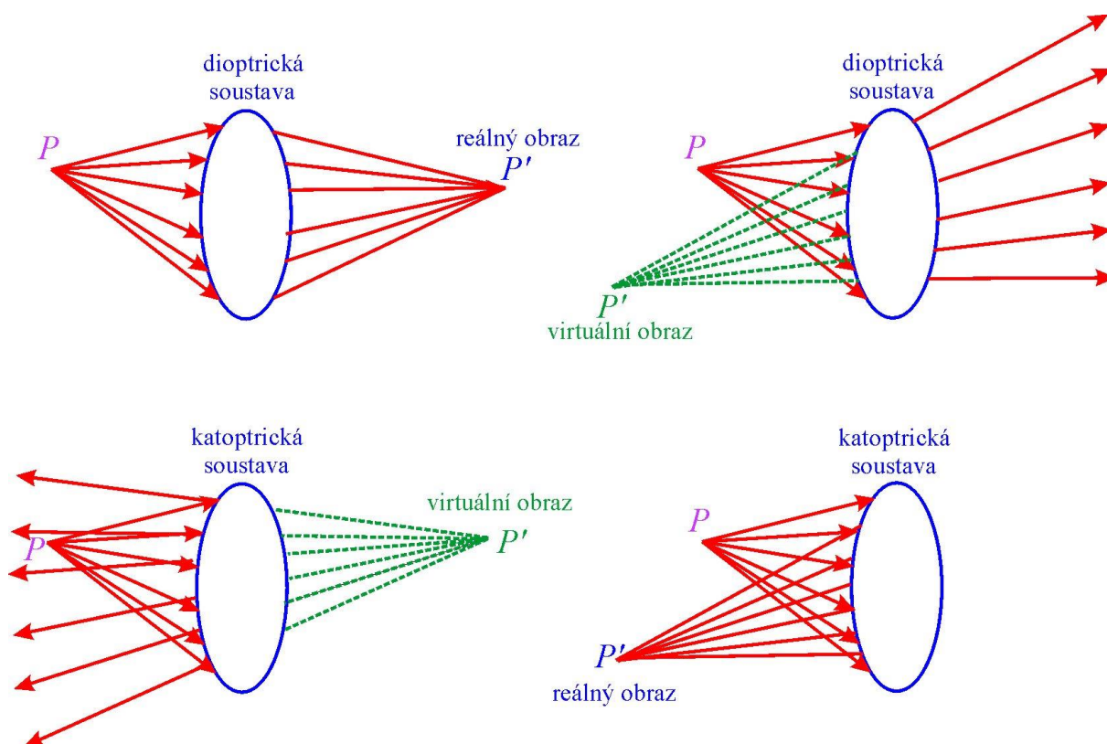
Obr. 8.11 Schématické znázornění reálného a virtuálního obrazu P' předmětového bodu P při zobrazování dioptrickou a katoptrickou soustavou s vyznačením homocentrických svazků
