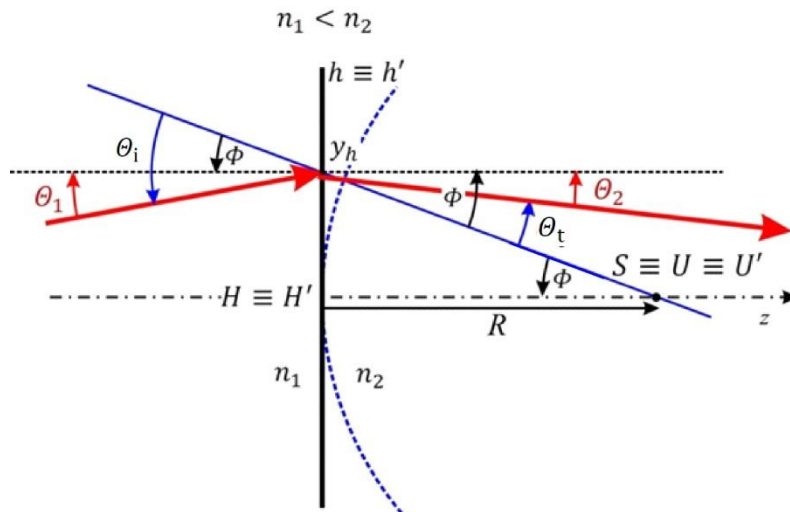
Obr. 8.20 Lom paprsku na kulové ploše v paraxiální aproximaci v tangenciální rovině. Rozměry a úhly zakreslené na obrázku z důvodu názornosti nesplňují požadavky paraxiální aproximace. Znaménka úhlů na obrázku:
