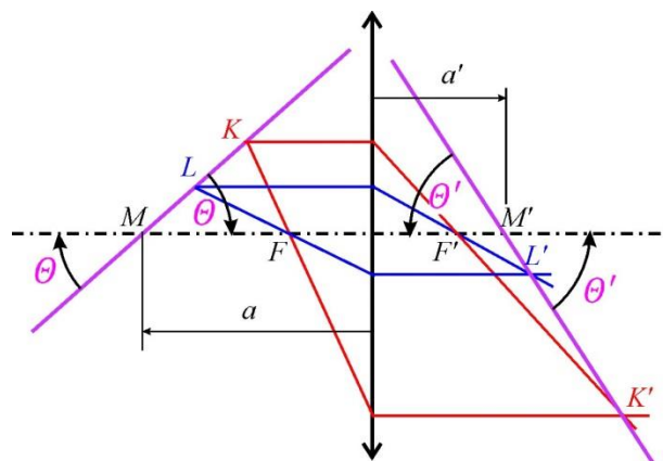
Obr. 8.28 Znárodnění úhlového zvětšení pro tenkou spojnou čočku ve vzduchu. Přímka KLM svírá s optickou osou úhel \theta (v obrázku záporný) a její obraz K'L'M' svírá úhel \theta' (v obrázku kladný).
