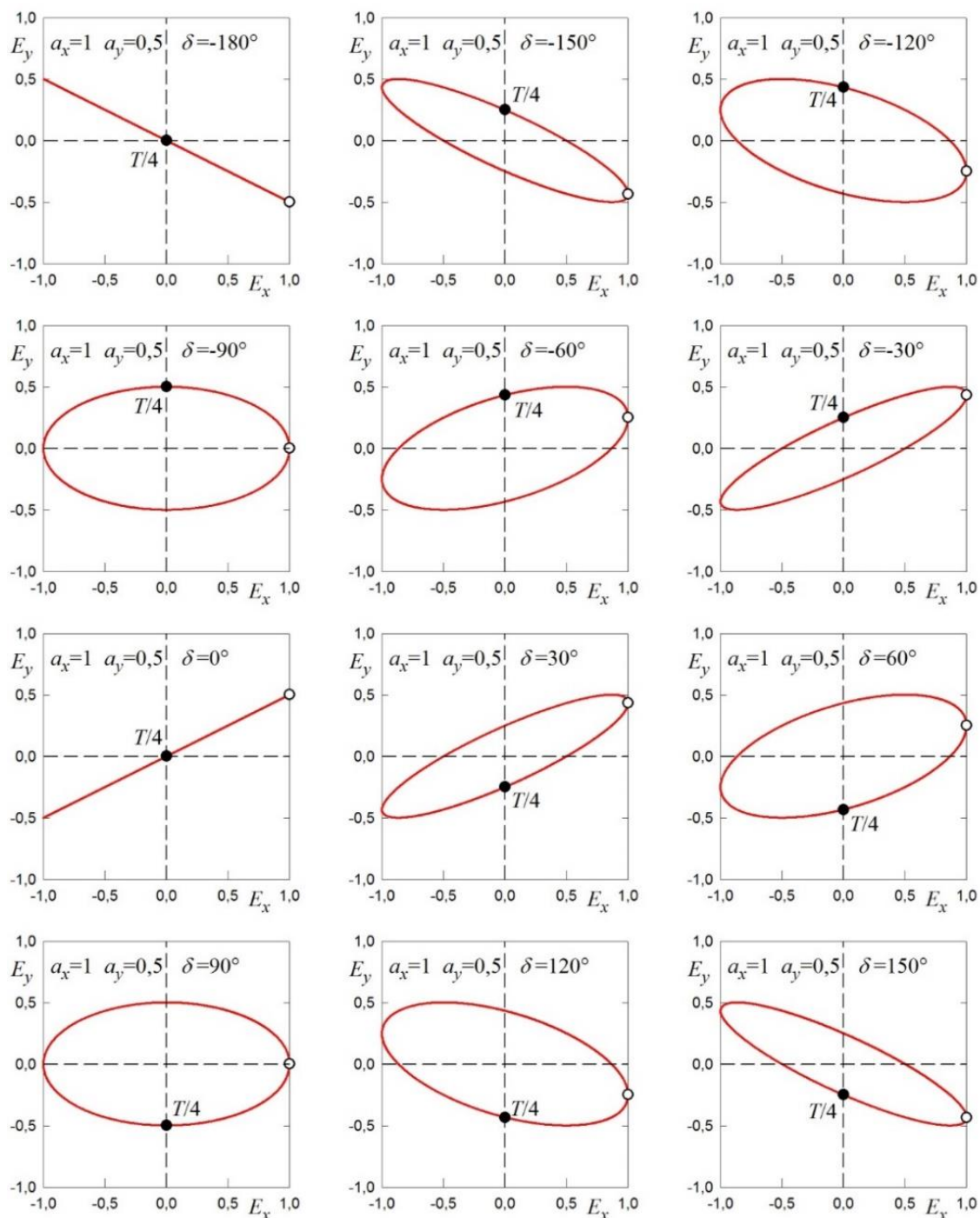
Obr. 2.7 Závislost tvaru polarizační elipsy na fázovém posuvu \delta . Pro všechny elipsy je E_x(t=0) = 1 . Pro E_y(t=T/4) > 0 je vlna levotočivá, pro E_y(t=T/4) < 0 je vlna pravotočivá. Podle rovnic (2.1) a (2.2) pro z = 0 .
