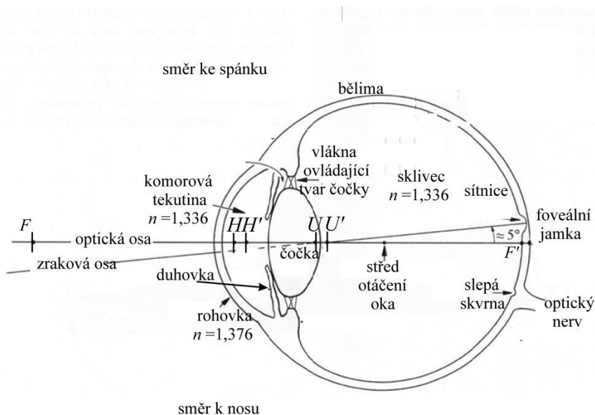
Obr. 8.30 Horizontální řez pravým okem. Nákres odpovídá oku zaostřenému na nekonečno.
