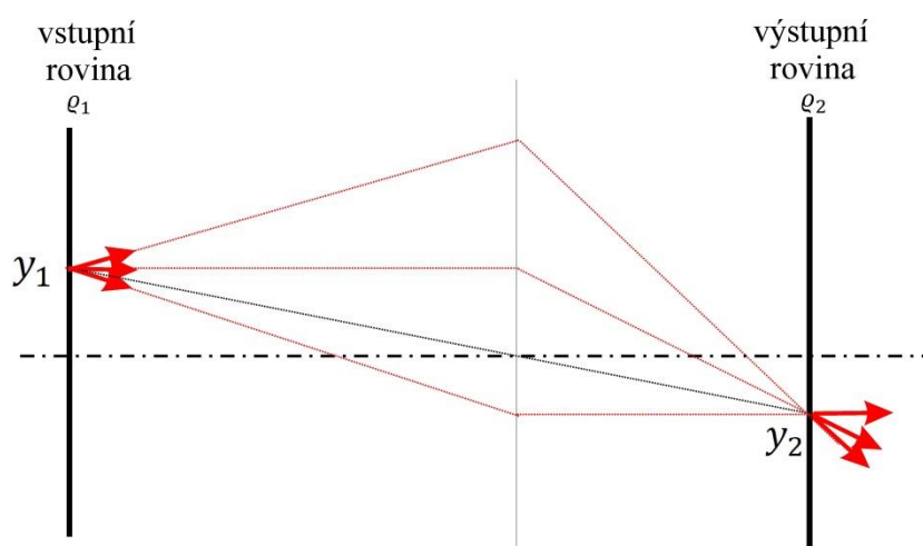
Obr. 8.17 Význam přenosové matice s B = 0 . Roviny q_1 a q_2 jsou konjugované.
