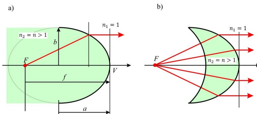
Obr. P8.5.2 Kolimace rozbíhavého svazku vycházejícího z bodového zdroje umístěného v ohnisku F . a) Základní geometrické uspořádání. b) Praktické provedení ve tvaru aplanaického menisku, kdy na první ploše (kulové se středem v F ) nedochází k lomu.
