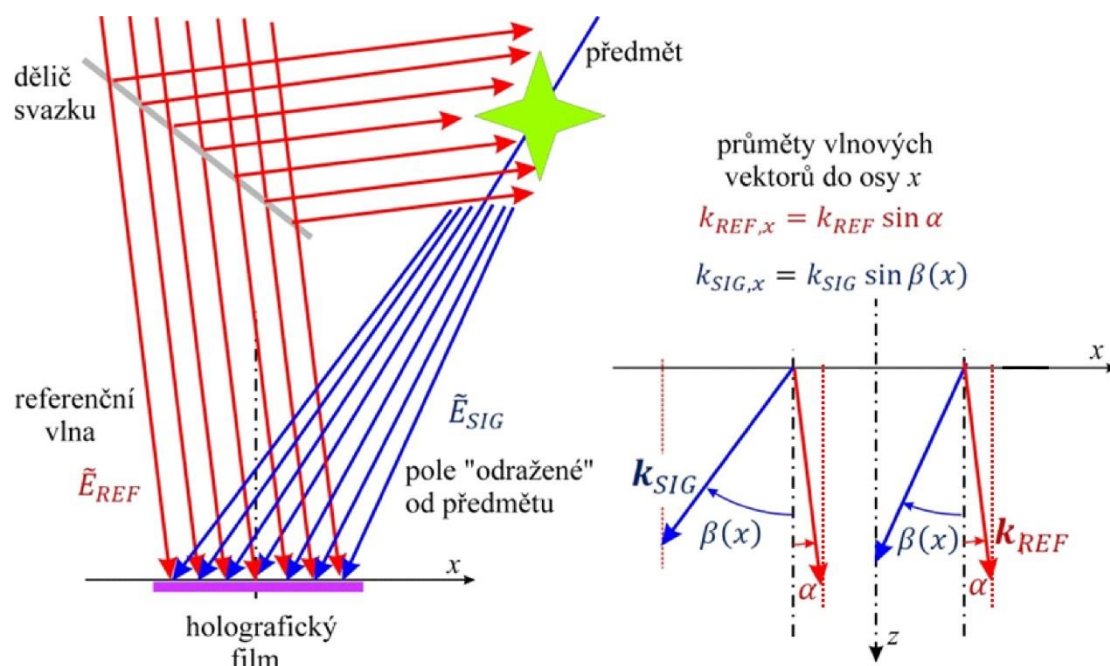
Obr. 6.30 Schéma pro holografický záznam a vlnové vektory referenční vlny a signálních vln
