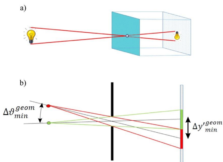
Obr. 8.39 Camera obscura a) Základní princip, b) minimální úhel rozlišení dvou bodů předmětu z hlediska geometrické optiky. V závislosti na velikosti vstupního otvoru přístroje je každý bod zobrazen jako kružnice. Minimální rozlišení je zde definováno podmínkou, aby se kružnice dvou sousedních rozlišitelných bodů nepřekrývaly.
