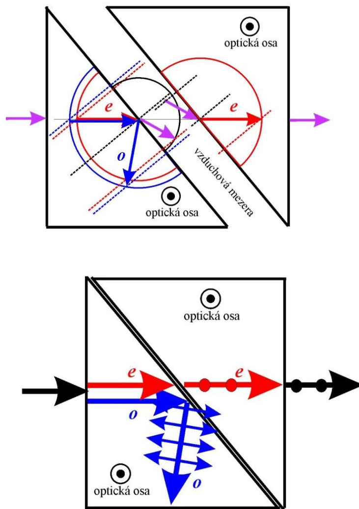
Obr. 10.10 Znázornění totálního odrazu řádného svazku na rozhraní krystal – vzduch pro vhodně zvolený úhel dopadu na toto rozhraní. V horní části obrázku jsou znázorněny vlnové vektory (včetně konstrukce lomu) a v dolní části obrázku příslušné polarizace. Průmět vlnového vektoru řádné vlny do roviny rozhraní je větší než průmět vlnového vektoru ve vzduchu. Nelze tedy splnit podmínku spojitosti (3.7) pro lomenou vlnu a dochází k totálnímu odrazu řádné vlny. Obrázek je nakreslen pro záporný krystal n_o > n_e a zhruba odpovídá realizaci s krystalem kalcitu. Část II polarizátoru již slouží jen pro „narovnání“ směru procházejícího svazku a v principu materiál části II ani nemusí být dvojlomný. Uspořádání se vzduchovou mezerou bývá označováno jako Glanův-Foucaultův polarizátor. Lepená verze (která musí brát v úvahu index lomu lepidla) se obvykle nazývá Glanův-Thompsonův polarizátor.
