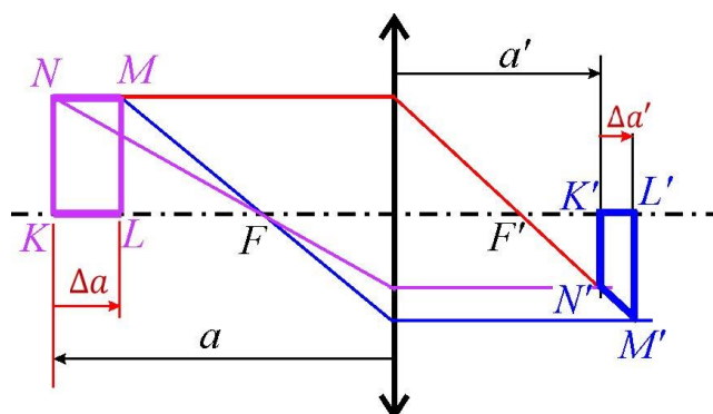
Obr. 8.29 Znázornění podélného zvětšení pro tenkou spojnou čočku ve vzduchu. Obrazem obdélníka KLMN o podélném rozměru \Delta a je lichoběžník K'L'M'N' podélného rozměru \Delta a' .
