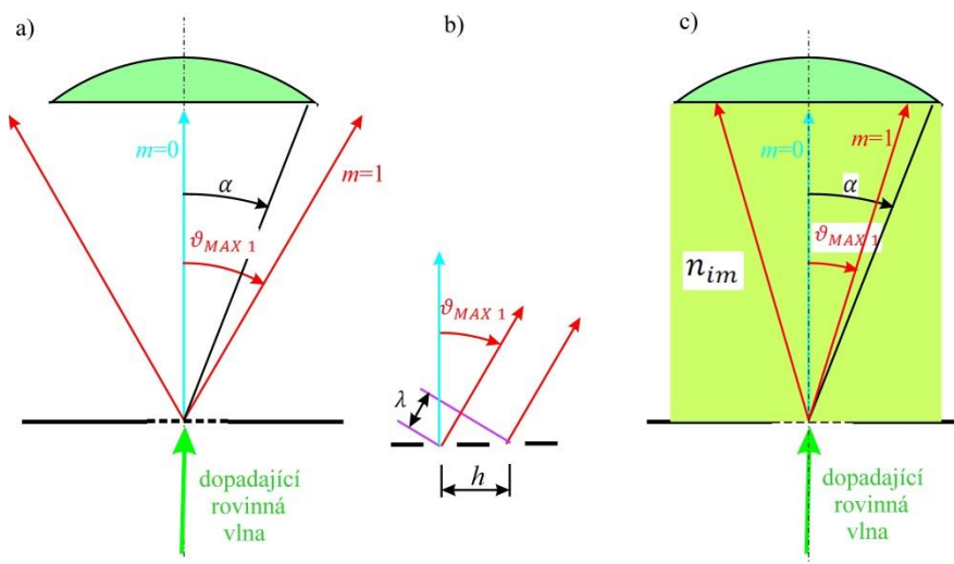
Obr. P8.6.2 Schématické znázornění Abbeova přístupu k popisu rozlišení mikroskopického objektivu. Vliv indexu lomu imerzní kapaliny spočívá ve změně vlnové délky \lambda_{im} = \lambda_0 / n_{im} .
