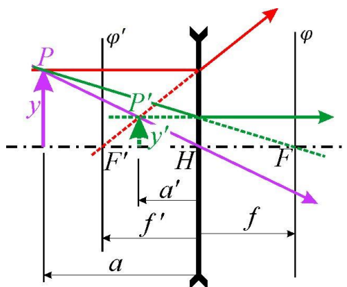
Obr. 8.25 e) Schéma zobrazení tenkou rozptylnou čočkou, f = -f' > 0 . Na obrázku jsou zakresleny paprsky (nebo jejich prodloužení) procházející ohnisky a paprsek procházející uzlovým bodem. Čárkovaně jsou vyznačena prodloužení reálných chodů paprsků: v levé části, „před čočkou“ je to prodloužení paprsku pro znázornění průchodu obrazovým ohniskem F' (červeně) a prodloužení paprsku pokračujícího „za čočkou“ rovnoběžně s osou (zeleně). V pravé části („za čočkou“) je čárkovaně naznačen původní směr zeleného paprsku směřujícího do předmětového ohniska F . Přitom je opět využito to, že v případě stejných indexů lomu na obou stranách čočky jsou uzlové body totožné s hlavními a navíc v aproximaci tenké čočky splývají obě hlavní roviny, tedy H \equiv U \equiv H' \equiv U' . Pro a < f' < 0 je obraz P' virtuální a přímý.
