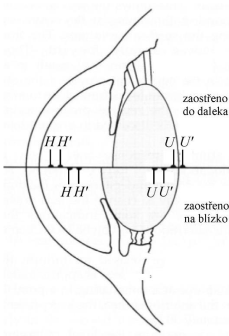
Obr. 8.31 Akomodace oka změnou tvaru oční čočky
