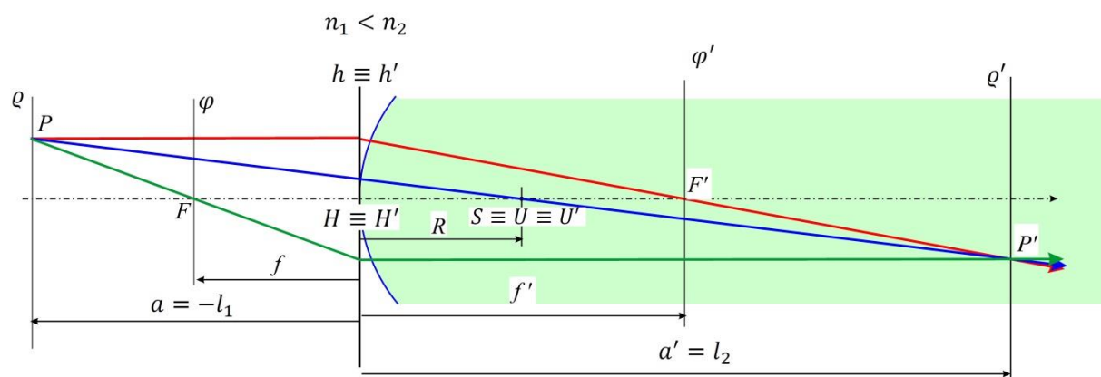
Obr. 8.21 Zobrazení jednou kulovou lomnou plochou v paraxiální aproximaci v meridiální rovině
