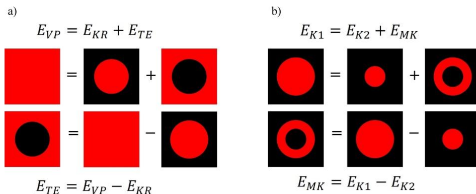
Obr. 6.9 a) Babinetův princip. Elektrické pole za nepropustným kruhovým terčíkem je rozdíl pole volného prostoru (žádná překážka) E_{VP} a pole za kruhovou aperturou E_{KR} téhož poloměru jako terčík.; b) Pole za aperturou tvořenou mezikružím E_{MK} v nepropustném stínítku lze spočítat jako rozdíl příspěvků od odpovídajících kruhových apertur E_{K1} - E_{K2} .
