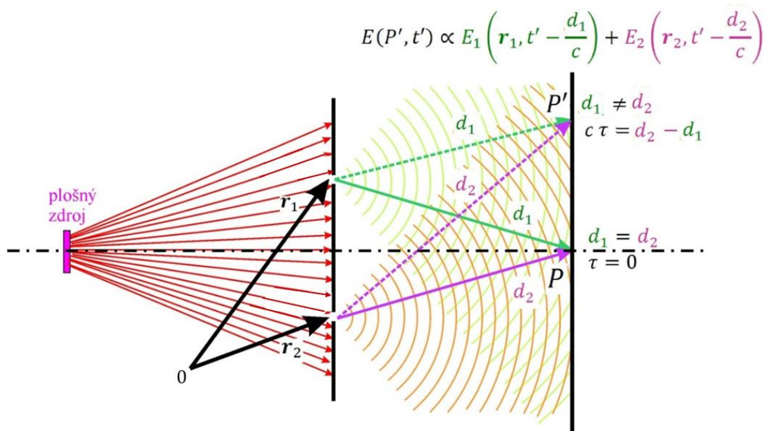
Obr. 7.2 Schéma pro zjišťování „čisté“ příčné ( \tau = 0 ) a „obecné“ ( \tau \neq 0 ) koherence polí E_1(\mathbf{r}_1, t) a E_2(\mathbf{r}_2, t) pomocí interference v Youngově uspořádání. Zdroj záření vyvolá ve štěrbině v místě \mathbf{r}_1 pole E_1(\mathbf{r}_1, t) a v místě \mathbf{r}_2 pole E_2(\mathbf{r}_2, t) . Výsledek interferenčního experimentu v bodě P' ukazuje korelaci polí v místech \mathbf{r}_1 a \mathbf{r}_2 a v časech t a t + \tau , tj. ve stacionárním případě souvisí s korelační funkcí \tilde{I}_{12}(\mathbf{r}_1, \mathbf{r}_2, \tau) , kde \tau = \frac{1}{c}(d_2 - d_1) . Speciálně pro d_2 = d_1 (tj. v bodě P ) je \tau = 0 a výsledek interference souvisí s korelační funkcí \tilde{I}_{12}(\mathbf{r}_1, \mathbf{r}_2, 0) . Obrázek je nakreslen pro častý případ záření jednoho plošného zdroje složeného z navzájem nekoherentních bodových zdrojů, kdy každý jednotlivý zdroj je časově zcela koherentní. Postup pro stanovení příčné a obecné koherence je však obecný, tj. lze jej využít i pro libovolné složené pole vznikající v důsledku působení mnoha různých zdrojů záření v prostoru před štěrbinami.
