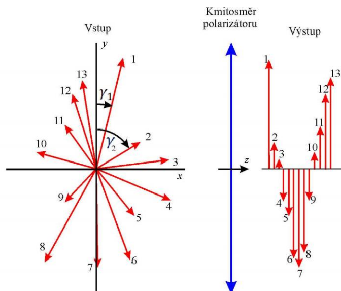
Obr. 2.11 Průchod nepolarizovaného světla polarizátorem. Vektor \mathbf{E} nabývá se stejnou pravděpodobností všech směrů v rovině xy . Úhly \gamma nabývají všech hodnot v intervalu \langle 0, 2\pi \rangle . Na obrázku jsou vyznačeny úhly \gamma_1 a \gamma_2 pro vektory \mathbf{E}_1(t) a \mathbf{E}_2(t) v nějakém časovém okamžiku. V obrázku je naznačen obecnější případ, kdy jednotlivé vlny mají různé amplitudy. Výpočet vedoucí k rovnici (2.18) předpokládá stejnou amplitudu vln \mathbf{E}_0 .
