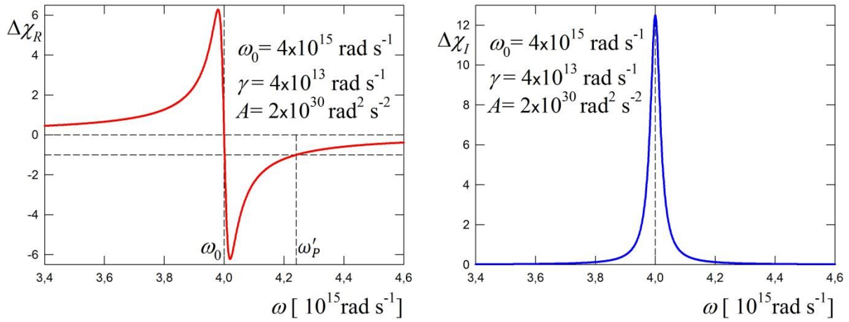
Obr. 12.4 Příspěvky k reálné a imaginární části susceptibility od jednoho typu lorentzovského oscilátoru. Kruhové frekvenci \omega_0 = 4 \times 10^{15} \text{ rad s}^{-1} odpovídá vlnová délka 471 nm.
