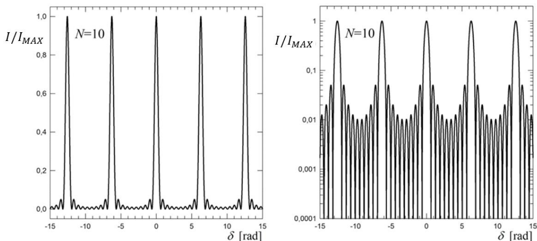
Obr. 4.16 Graf funkce \frac{\sin^2\left(N \frac{\delta}{2}\right)}{N^2 \sin^2\left(\frac{\delta}{2}\right)} pro N = 10 . Funkce je periodická s periodou 2\pi .
