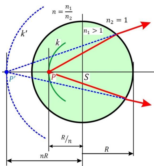
Obr. 8.9 Descartova kulová lomná plocha zobrazující stigmaticky vnitřní kulovou plochu k na vnější plochu k' . V uvedeném případě je obraz virtuální.
