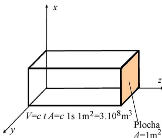
Obr.1.4 Objem V = ctA , ve kterém se nachází záření, které projde plochou 1\text{m}^2 za 1\text{s} . Postupná rovinná vlna se šíří ve směru osy z .
