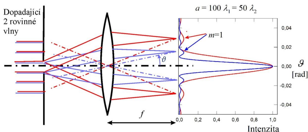
Obr. 6.23 Schématické znázornění Fraunhoferovy difrakce na obdélníkové apertuře (štěrbíně) šířky a v řezu y = 0 s fokusační čočkou. Vlnové délky kolmo dopadajících rovinných vln jsou \lambda_1 = a/100 a \lambda_2 = a/50 . Úhel \theta je v obrázku zveličen. Pro první vedlejší maximum difrakce na 1 štěrbíně je pro uvedené hodnoty \theta_{\lambda_1, m_{1st}=1} \cong 0,0143 \text{ rad} \cong 0,82^\circ a \theta_{\lambda_2, m_{1st}=1} \cong 0,0286 \text{ rad} \cong 1,64^\circ . Červená ( \lambda_2 ) a modrá ( \lambda_1 ) barva v tomto obrázku (na rozdíl od předchozích obrázků) reprezentují různé vlnové délky světla.
