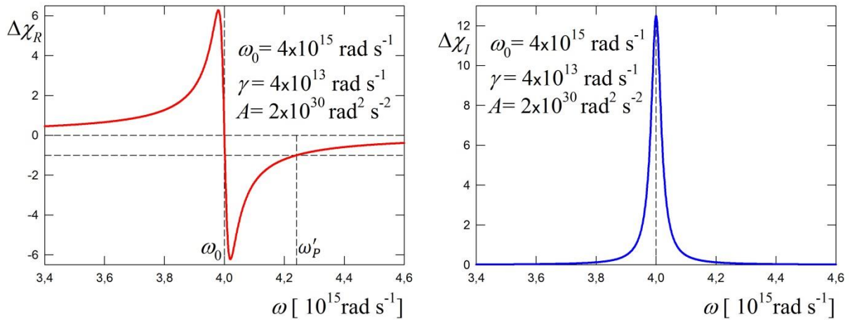
Obr. 12.4 Příspěvky k reálné a imaginární části susceptibility od jednoho typu lorentzovského oscilátoru. Kruhové frekvenci \omega_0 = 4 \times 10^{15} \text{ rad s}^{-1} odpovídá vlnová délka 471 nm.
