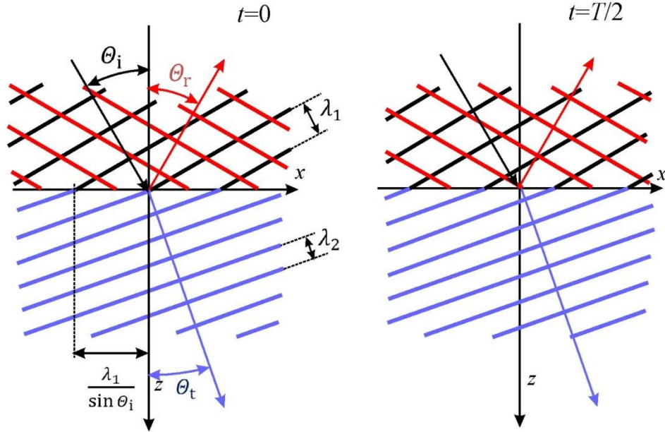
Obr. 3.3 Znázornění navazování vlnoploch při odrazu a lomu. Situace odpovídá odrazu na opticky hustším prostředí pro úhel dopadu \theta_i = 30^\circ . Zakreslena jsou kladná maxima elektrických polí: černě dopadající vlna, červeně odražená vlna a modře lomená vlna. Posun vlnoploch za čas t = \frac{T}{2} = \frac{\pi}{\omega} v pravé části obrázku odpovídá polovině periody \frac{\Lambda_x}{2} = \frac{\lambda_1}{2 \sin \theta_i} . Maxima odražené vlny jsou v tomto případě (odraz na neabsorbujícím opticky hustším prostředí) posunuta o \frac{\Lambda_x}{2} vůči maximům vlny dopadající i lomené. To odpovídá fázovému posunu vlny odražené vůči vlně dopadající o fázový úhel \pi . Bude odvozeno v kapitole 3.2.4.
