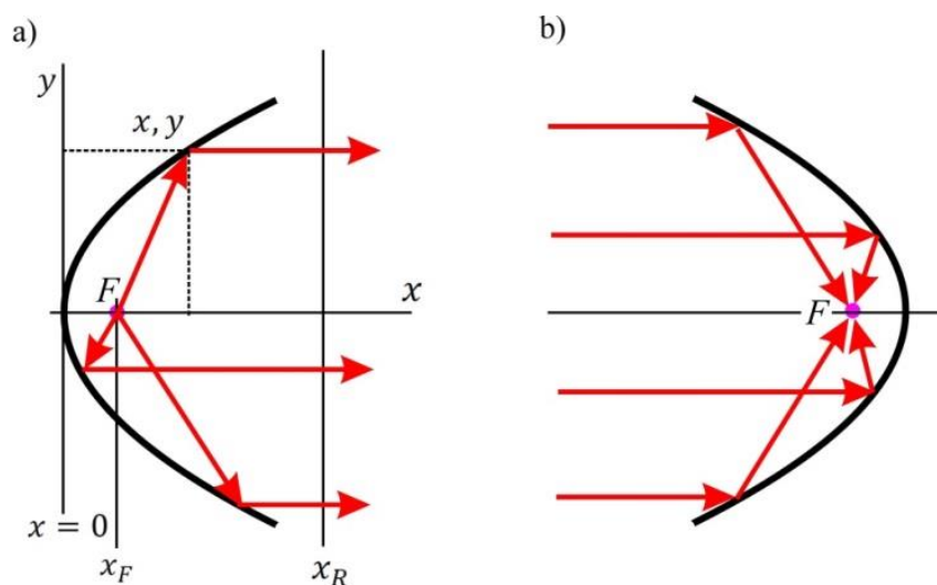
Obr. P8.5.7 a) Kolimace homocentrického svazku paprsků odrazem na ploše paraboloidu. b) Fokuzace rovnoběžného svazku paprsků.
