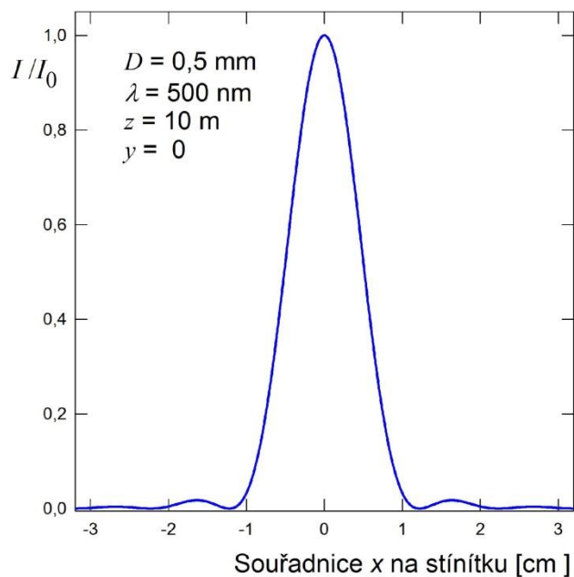
Obr. 6.18 Normované rozložení intenzity difraktovaného světla při Fraunhoferově difrakci na kruhovém otvoru průměru D = 0,5 \text{ mm} a s dalšími uvedenými parametry.
