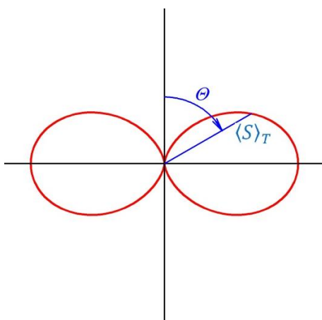
Obr. 1.6 Řez vyzářovacím diagramem Hertzova dipólu. Délka úsečky ve směru určeném úhlem \theta je úměrná střední hodnotě velikosti Poyntingova vektoru do tohoto směru. Diagram je osově symetrický kolem „svislé“ osy ( \theta = 0 ).
