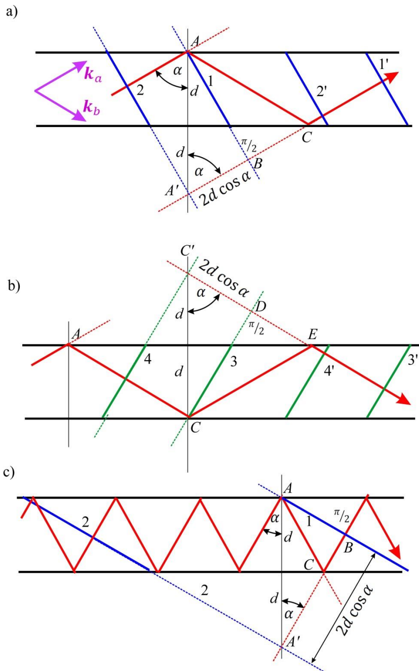
Obr. 9.3 a) Geometrická konstrukce k určení dráhového rozdílu mezi vlnoplochami procházejícími body A a A' . Paprsky jsou kresleny červeně a vlnoplochy modře. Vlnoplochy 1 a 2 jsou zakresleny pro jeden okamžik, vlnoplochy 1' a 2' znázorňují jejich polohu v pozdějším čase. Trojúhelník ABA' je pravoúhlý s přeponou AA' délky 2d a odvěsna A'B má délku 2d \cos \alpha . Nakresleno pro případ velkého úhlu \alpha a paprsky směřující k horní části obrázku. b) Určení dráhového rozdílu mezi vlnoplochami procházejícími body C a C' . Paprsky jsou kresleny červeně a vlnoplochy zeleně. Pro případ velkého úhlu \alpha a paprsky směřující k dolní části obrázku. c) Pro malý úhel \alpha , který ovšem ještě musí splňovat podmínku totálního odrazu. V obrázku a) jsou zakresleny i vlnové vektory interferujících rovinných vln: \mathbf{k}_a se vztahuje k modrým vlnoplochám na obr. a) a \mathbf{k}_b se vztahuje k zeleným vlnoplochám na obr. b).
