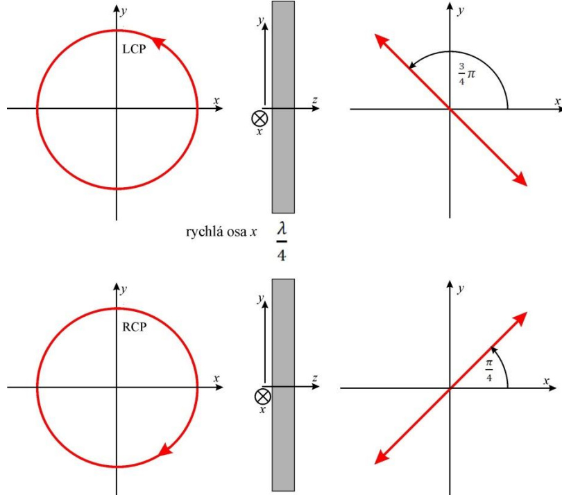
Obr. 2.14 Schématické znázornění působení čtvrtvlnové destičky na kruhově polarizovanou vlnu.
