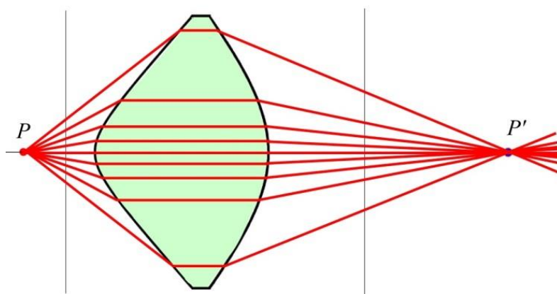
Obr. P8.5.5 Příklad spojně čočky tvořené dvěma lomnými plochami hyperboloidů, která stigmaticky zobrazuje bod P do bodu P' . V čočce se šíří rovnoběžný svazek.
