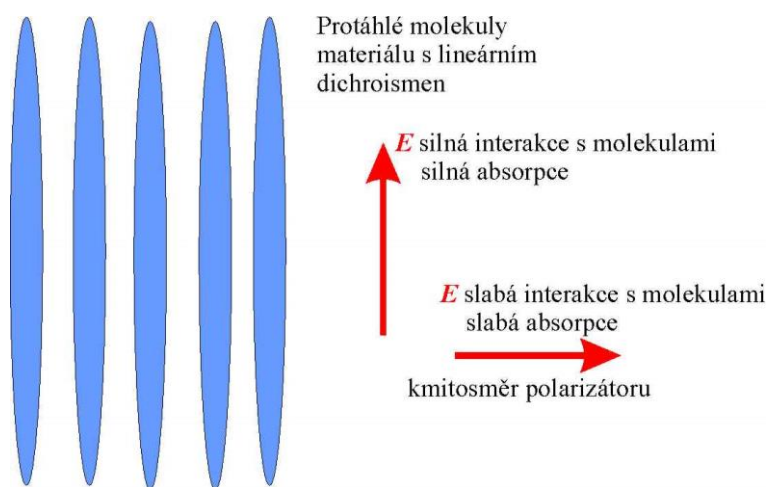
Obr. 2.8 Schématické znázornění principu dichroického polarizátoru
