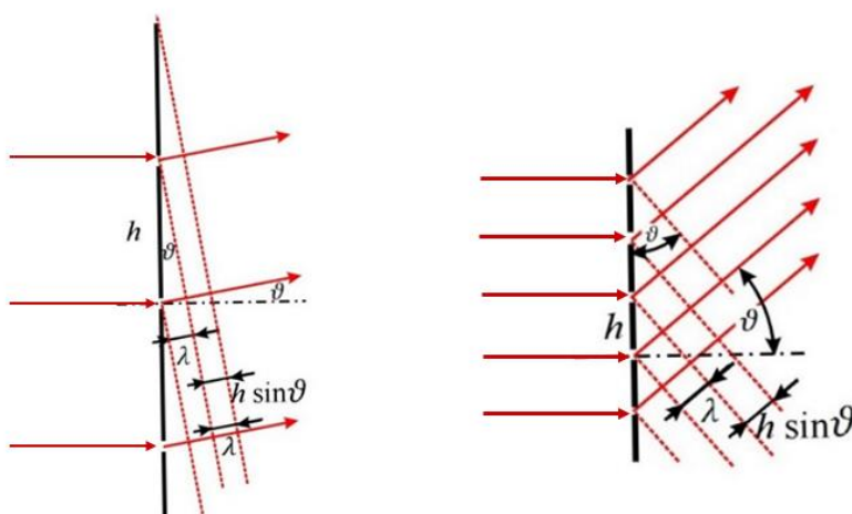
Obr 6.26 Souvislost mezi úhlem \vartheta_{MAX\ 1} a vzdáleností štěrbin. Pro velká h je dosaženo podmínky maxima h \sin \vartheta_{MAX\ 1} = \lambda pro m = 1 při menších úhlech \vartheta než pro malá h .
