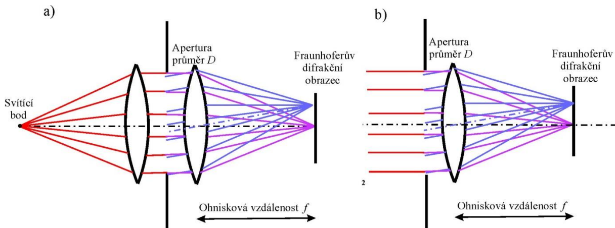
Obr. 6.20 Model zobrazení monochromatického svítícího bodu ideální optickou soustavou při aperturní cloně průměru D ; a) blízký bod, kulová vlna je před dopadem na aperturu kolimována čočkou na rovinnou vlnu (rovnoběžné paprsky). f_2 je ohnisková vzdálenost 2. části zobrazovací soustavy; b) velmi vzdálený bod, na aperturu dopadá rovinná vlna
