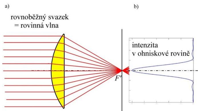
Obr. P8.4.1 a) Znáznornění fokusace rovnoběžného svazku v modelu paprskové optiky. b) Rozložení intenzity v ohniskové rovině ve skalárním modelu Fraunhoferovy difrakce, viz též obr. 6.18.
