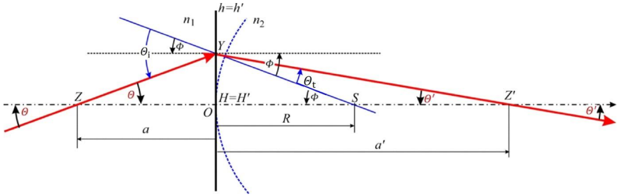
Obr. 8.22 K odvození Abbeova invariantu paraxiální optiky
