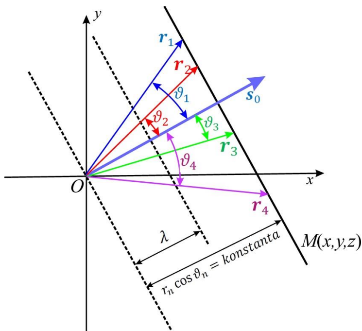
Obr. 1.1 Znáornění řezů rovinných vlnoploch pro vlnu s vlnovým vektorem \mathbf{k} = (k_x, k_y, 0) = k \mathbf{s}_0 . Čárkovaně je zakreslen řez vlnoplochou procházející počátkem souřadné soustavy a řez další vlnoplochou vzdálenou od počátku o vlnovou délku \lambda . Barevně jsou zakresleny čtyři polohové vektory reprezentující obecný polohový vektor bodu na vlnoploše M . Vzdálenosti r_i různých bodů vlnoplochy M od počátku v jednom libovolném čase splňují podmínku \mathbf{s}_0 \cdot \mathbf{r}_i = s_{0x}x_i + s_{0y}y_i = r_i \cos \vartheta_i = vt . Vlnová délka je \lambda = vT , T je doba kmitu.
