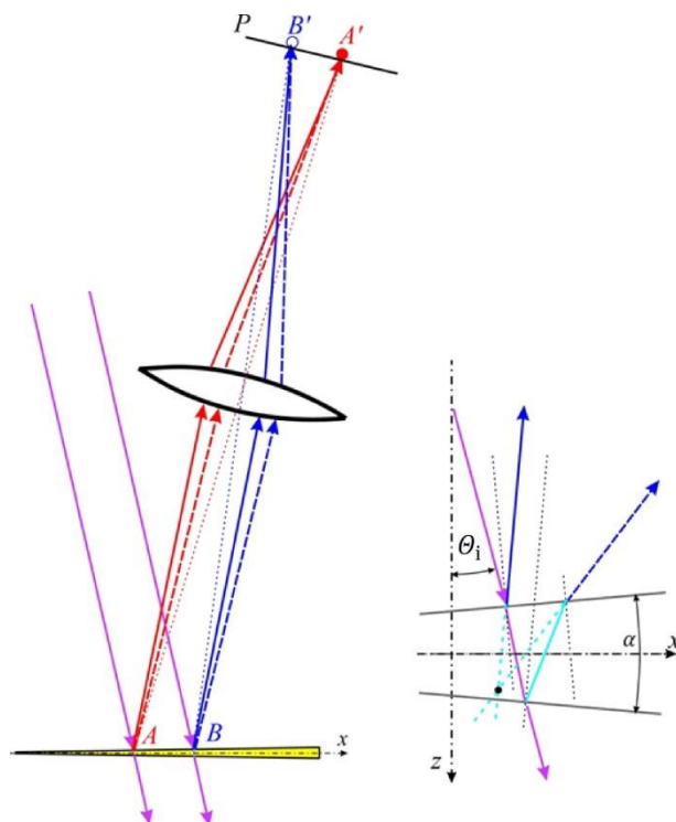
Obr. 4.15 Paprskový model interference na tenkém klínu. O tom, zda se v místě pozorování A' objeví interferenční proužky maximální intenzity nebo intenzity minimální, rozhoduje splnění podmínek v místě A pro fázový rozdíl mezi přímo odraženou vlnou (plné čáry) a vlnou odraženou na spodní straně klínu (čárkované čáry). Právě v místě A' dojde k interferenci částí vlnoploch vln vycházejících z oblasti kolem bodu A a odvozených od původního paprsku dopadajícího do oblasti A . Analogická situace nastává pro jiné zvolené místo na klínu B a místo pozorování B' .
