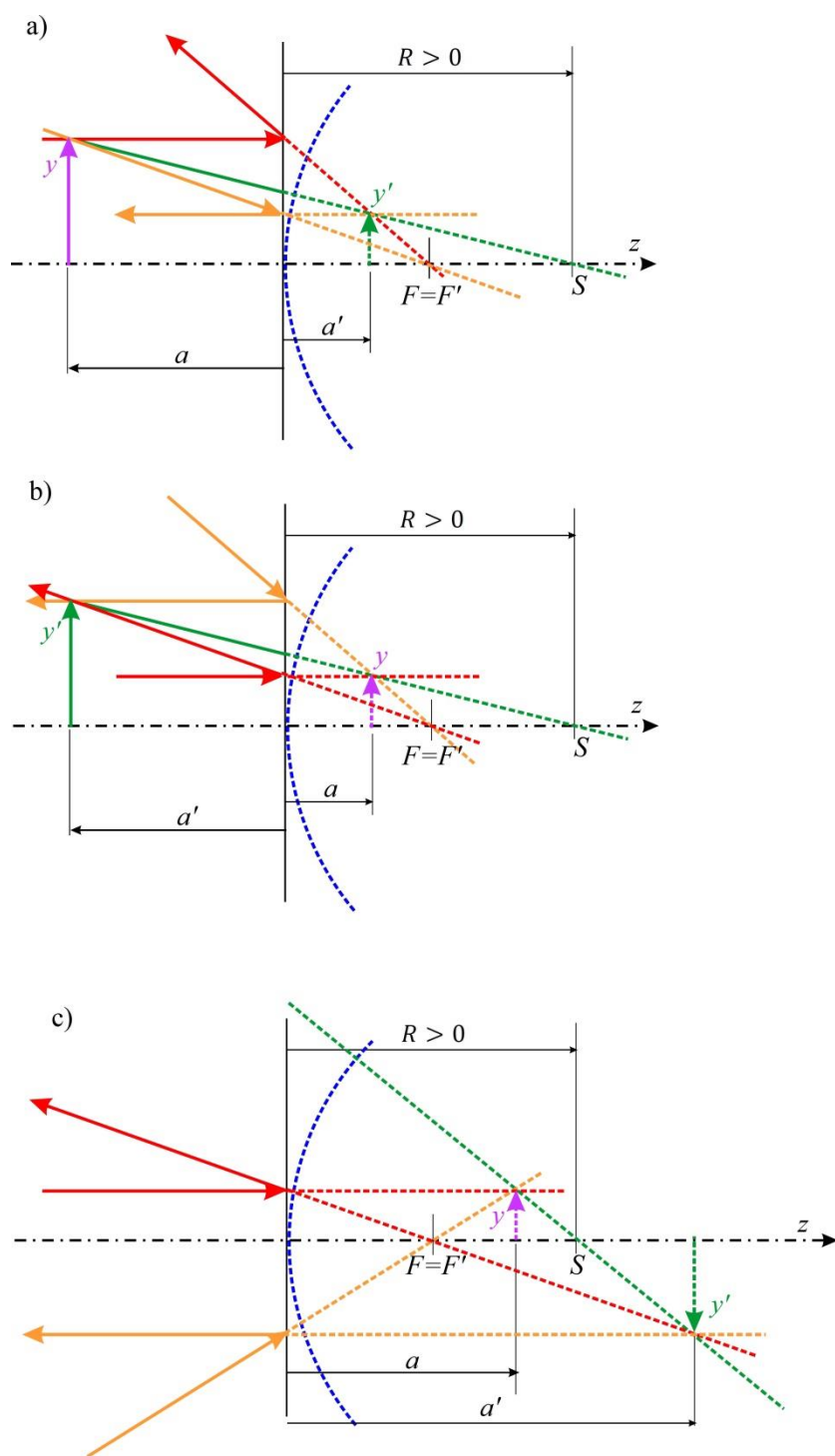
Obr. P.8.7.2 Zobrazení vypuklým (konvexním) zrcadlem v paraxiální aproximaci. a) Obraz (zeleně) předmětu před zrcadlem se nachází za zrcadlem a je virtuální a přímý. b) Obrácený chod paprsků oproti případu a), kdy virtuální předmět je umístěn mezi odraznou plochou a ohniskem. Jeho obraz je reálný a přímý. c) Virtuální předmět je za ohniskem a jeho obraz je virtuální a převrácený.
