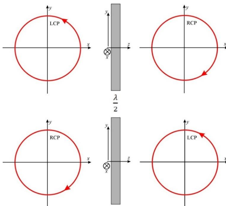
Obr. 2.17 Schématické znázornění působení polovlnové destičky na kruhově polarizované světlo
