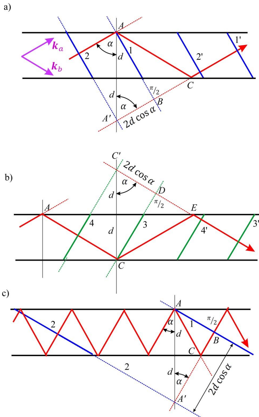
Obr. 9.3 a) Geometrická konstrukce k určení dráhového rozdílu mezi vlnoplochami procházejícími body A a A'. Paprsky jsou kresleny červeně a vlnoplochy modře. Vlnoplochy 1 a 2 jsou zakresleny pro jeden okamžik, vlnoplochy 1' a 2' znázorňují jejich polohu v pozdějším čase. Trojúhelník ABA' je pravoúhlý s přeponou AA' délky 2d a odvěsna A'B má délku 2d \cos \alpha . Nakresleno pro případ velkého úhlu \alpha a paprsky směřující k horní části obrázku. b) Určení dráhového rozdílu mezi vlnoplochami procházejícími body C a C'. Paprsky jsou kresleny červeně a vlnoplochy zeleně. Pro případ velkého úhlu \alpha a paprsky směřující k dolní části obrázku. c) Pro malý úhel \alpha , který ovšem ještě musí splňovat podmínku totálního odrazu. V obrázku a) jsou zakresleny i vlnové vektory interferujících rovinných vln: k_a se vztahuje k modrým vlnoplochám na obr. a) a k_b se vztahuje k zeleným vlnoplochám na obr. b).
