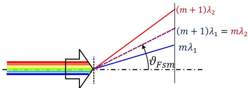
Obr. 6.30 Volný spektrální interval. Na difrakční mřížku dopadá světlo v intervalu vlnových délek (\lambda_1, \lambda_2) . Podmínkou dobrého zobrazení je, že difrakční úhel paprsku s vlnovou délkou \lambda_2 difraktovaného v m -tém řádu nepřesáhne difrakční úhel paprsku s vlnovou délkou \lambda_1 difraktovaného v m + 1 řádu.
