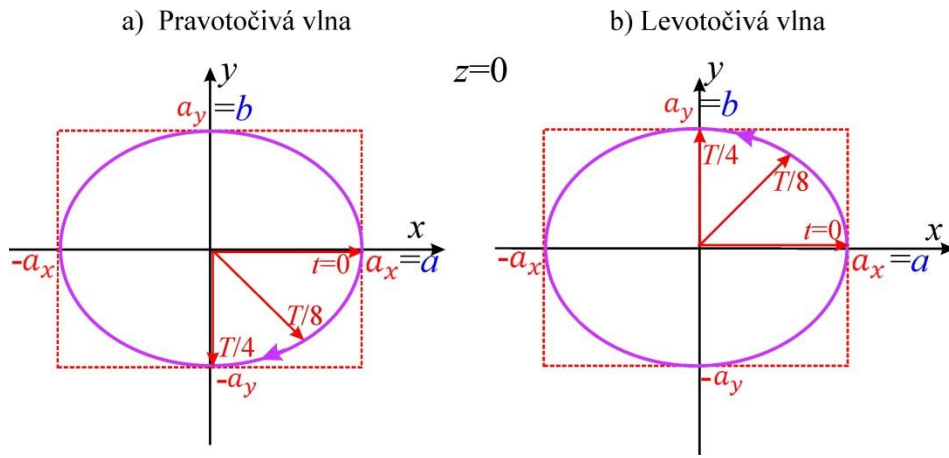
Obr. 2.4 a) Pravotočivá, elipticky polarizovaná vlna, pro kterou platí \delta = \frac{\pi}{2} , a = a_x > a_y = b . Pohled proti směru šíření v jedné rovině prostoru (zvoleno z = 0 ). Koncový bod vektoru \mathbf{E} obíhá elipsu po směru hodinových ručiček. b) Levotočivá, elipticky polarizovaná vlna, pro kterou platí a = a_x > a_y = b , \delta = -\frac{\pi}{2} . Koncový bod vektoru \mathbf{E} obíhá elipsu proti směru hodinových ručiček.
