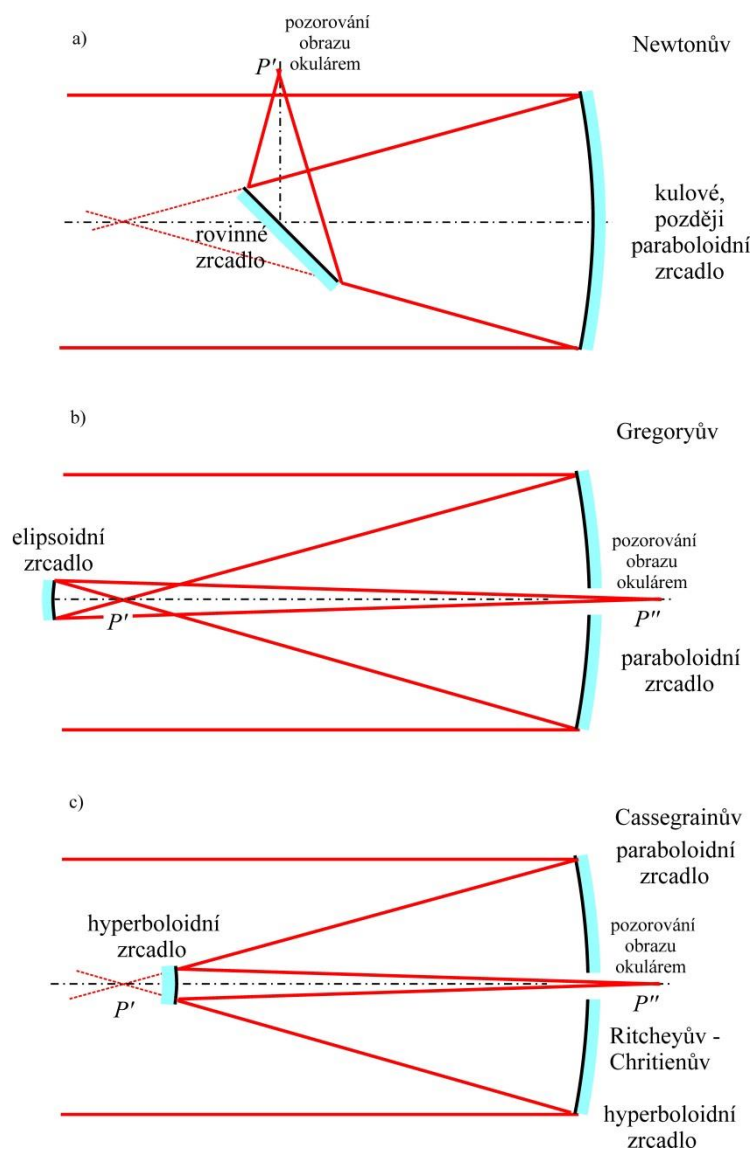
Obr. 8.38 Schémata základních typů zrcadlových teleskopů. a) Newtonův teleskop využíval v první verzi (1668) fokuzace kulovou odraznou plochou, v pozdějších verzích paraboloidní plochou. Obraz bylo možno sledovat okulárem. b) Gregoryův teleskop (první realizace podle Gregoryova návrhu Hook 1673) jako primární zrcadlo používá paraboloid vytvářející reálný obraz P' a ten je zobrazen do reálného obrazu P'' . c) Cassegrainův systém používá k zobrazení virtuálního bodu P' pomocí reflexní hyperboloidní plochy do reálného P'' . Dnes nejvíce používaný systém pro „velké“ dalekohledy vychází z hyperboloidní plochy primárního zrcadla a dále je shodný s Cassegrainovým schématem. Je pojmenován podle jmen George Willis Ritchey a Henri Jacques Chrétien, Konstrukce byla realizována kolem roku 1910.
