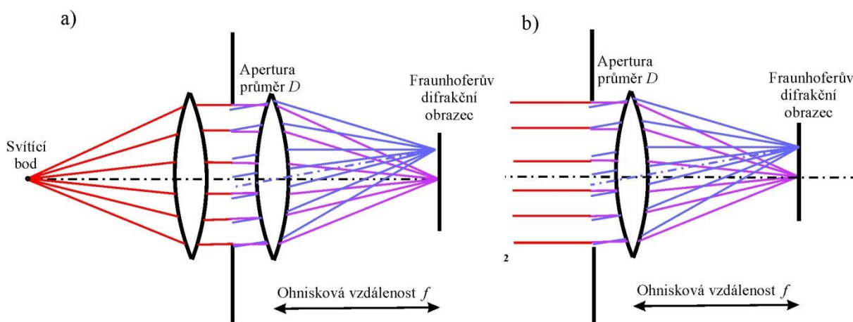
Obr. 6.20 Model zobrazení monochromaticky svítícího bodu ideální optickou soustavou při aperturní cloně průměru D ; a) blízký bod, kulová vlna je před dopadem na aperturu kolimována čočkou na rovinnou vlnu (rovnoběžné paprsky). f_2 je ohnisková vzdálenost 2. části zobrazovací soustavy; b) velmi vzdálený bod, na aperturu dopadá rovinná vlna
