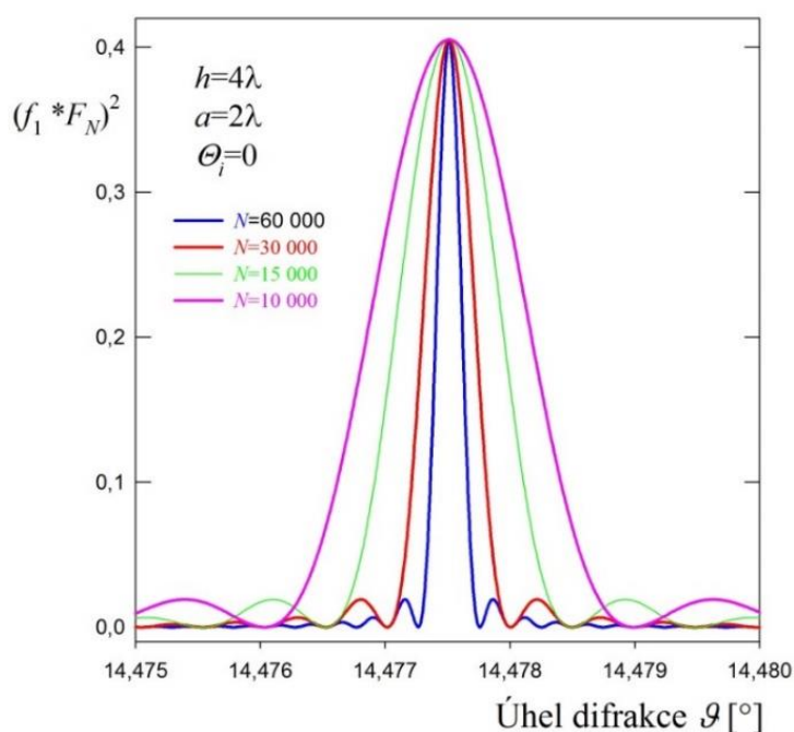
Obr. 6.29 Modelová závislost normované intenzity difraktované vlny (f_1 F_N)^2 v okolí 1. hlavního maxima m = 1 pro mřížky s počtem štěrbin N = 60\,000, 30\,000, 15\,000 a 10\,000 .
