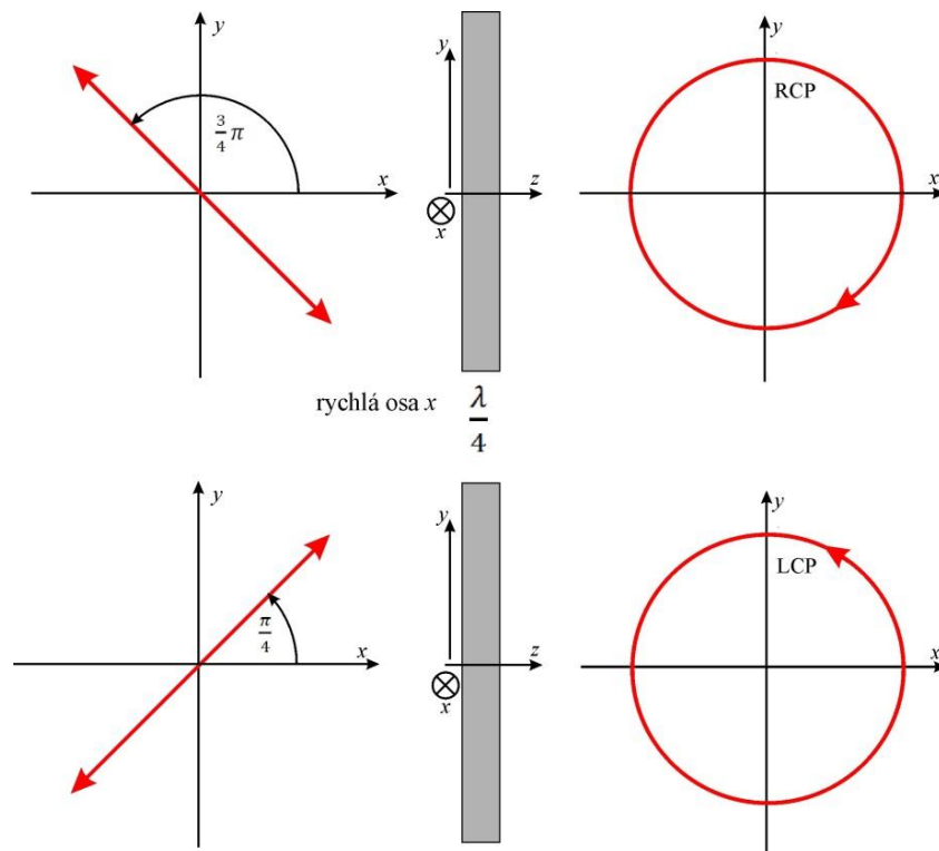
Obr. 2.15 Schématické znázornění působení čtvrtvlnové destičky na lineárně polarizovanou vlnu.
