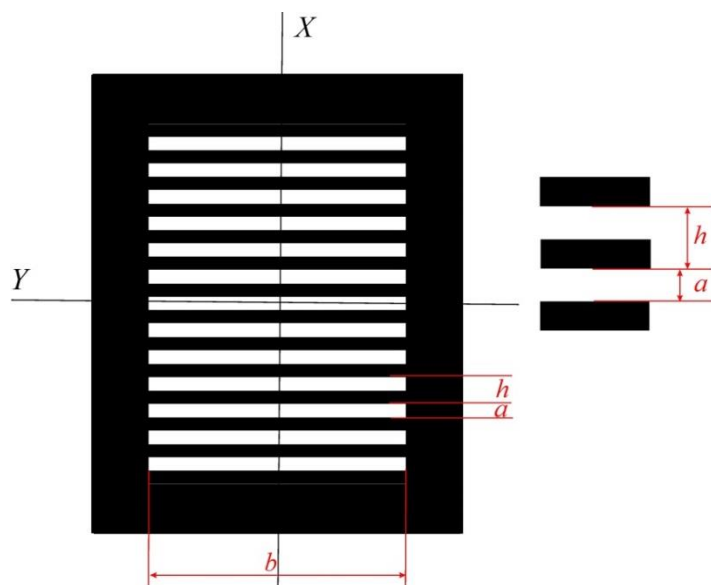
Obr. 6.24 Amplitudová mřížka na průchod tvořená periodicky umístěnými obdélníkovými štěrbinami v neprůhledném stínítku
