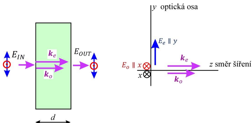
Obr. 2.12 Uspořádání pro vysvětlení principu fázové destičky. Je zakreslen případ kladného krystalu, tj. n_e > n_o , např. křemen. Pak je fázová rychlost řádné vlny v_x = v_o větší než fázová rychlost mimořádné vlny v_y = v_e a osu x označíme jako „rychlá osa“.
