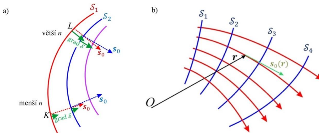
Obr. 8.4 a) Znázornění řezů plochami eikonálů o hodnotách \mathcal{S}_1 (červeně) a \mathcal{S}_2 (modře). Zeleně jsou zakresleny gradienty eikonálu v místech K a L. V místě K jsou \mathcal{S}_1 a \mathcal{S}_2 od sebe vzdálenější než v místě L, takže gradient je v K menší než v L. To je přímo určeno indexem lomu n , který je v oblasti K menší než v oblasti L. Směry paprsků \mathbf{s}_0 jsou rovnoběžné s \text{grad } \mathcal{S} ; v obrázku jsou z důvodu přehlednosti poněkud posunuty. Směry paprsků jsou stáčeny do oblasti prostoru s větším indexem lomu. b) Řezy plochami konstantních eikonálů (modře) a paprsky (červeně) pro jiné prostorové rozložení indexu lomu než v obr. a). Tečna \mathbf{s}_0(\mathbf{r}) k paprsku v místě \mathbf{r} je naznačena zeleně.
