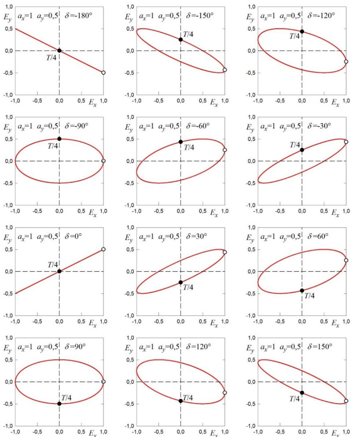
Obr. 2.6 Závislost tvaru polarizační elipsy na fázovém posuvu \delta . Pro všechny elipsy je E_x(t=0) = 1 . Pro E_y(t=T/4) > 0 je vlna levotočivá, pro E_y(t=T/4) < 0 je vlna pravotočivá. Podle rovnic (2.1) a (2.2) pro z = 0 .
