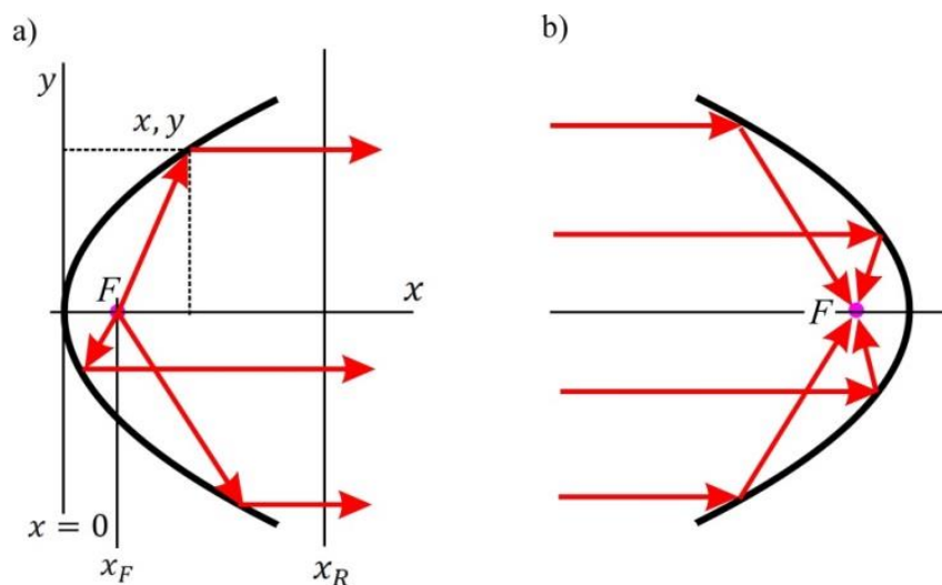
Obr. P8.5.7 a) Kolimace homocentrického svazku paprsků odrazem na ploše paraboloidu. b) Fokuzace rovnoběžného svazku paprsků.
