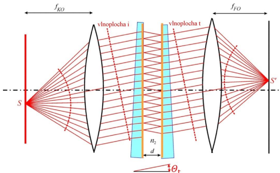
Obr. 4.21 Fabryův-Pérotův interferometr se vstupující jednou rovinnou vlnou. Intenzita obrazu S' bodového zdroje S je modulována funkcí danou vztahem (4.38). O tom, zda bude obraz intenzivní nebo naopak temný, rozhoduje při pevném nastavení d, n_2 úhel \theta_t , tedy poloha bodu S . Interferometr lze ladit právě mechanickou změnou d (např. piezoelektricky) nebo indexu lomu n_2 (např. tlakem plynu v prostoru mezi deskami). Vzhledem k osové symetrii jsou při „rozsvícení“ mnoha bodů ve fokální rovině kolimátoru pozorovány kroužky stejného sklonu. Poloha intenzitních maxim je podobná jako u jiných interferometrů, ale velmi podstatný rozdíl je v jejich vysoké ostrosti pro kvazimonochromatické záření s velmi úzkou spektrální čarou.
