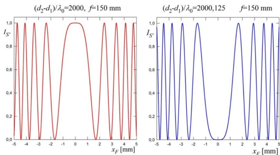
Obr. 4.7 Průběh intenzity záření I_{S'}(x_F, y_F) v ohniskové rovině pro uvedené parametry ukazující intenzitu kroužků stejného sklonu
