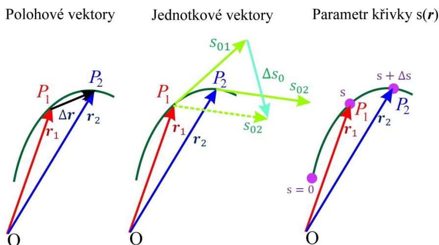
Obr. 8.3 Zobrazení základních pojmů spojených se zavedením paprsku jako prostorové křivky. Poloha bodů, kterými paprsek prochází, je určena polohovými vektory \mathbf{r}_1 a \mathbf{r}_2 . Jednotkové vektory ve směru tečen k paprsku jsou \mathbf{s}_0 . Délka dráhy podél paprsku je určena skalární veličinou – parametrem s .
