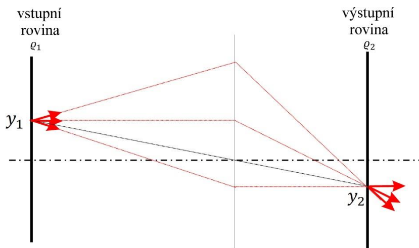
Obr. 8.17 Význam přenosové matice s B = 0 . Roviny \varrho_1 a \varrho_2 jsou konjugované.
