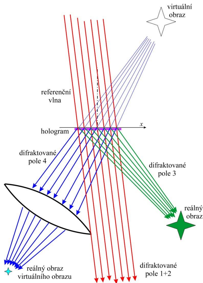
Obr. 6.36 Zobrazení holografického záznamu. Exponovaný hologram je osvětlen referenční vlnou o stejné frekvenci a směru, jaká byla použita při expozici. Nejdůležitější je difraktované pole 4, které vytváří virtuální obraz v místě původního předmětu. Za použití spojné optiky lze tento virtuální obraz převést na reálný. V případě vizuálního pozorování je tímto optickým systémem rohovka a čočka oka a reálný obraz vzniká na sítnici. Pozorovatel vidí obraz zaznamenané scény ve směru, ve kterém dopadala na film signální vlna při expozici.
