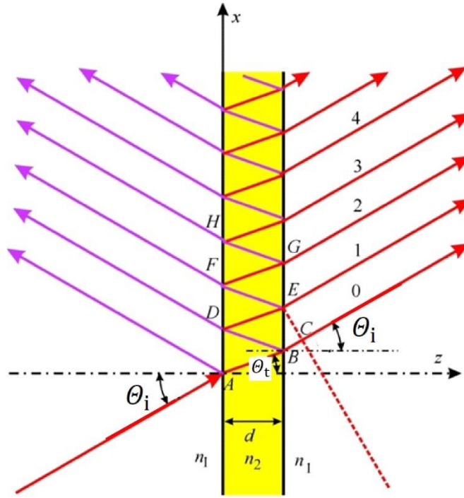
Obr. 4.17 Paprskový model mnohonásobných odrazů v planoparalelní dielektrické desce Vlna lomená v bodě G (vlna 2)
