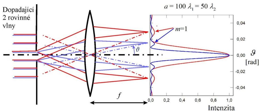
Obr. 6.23 Schématické znázornění Fraunhoferovy difrakce na obdélníkové apertuře (štěrbině) šířky a v řezu y = 0 s fokusační čočkou. Vlnové délky kolmo dopadajících
