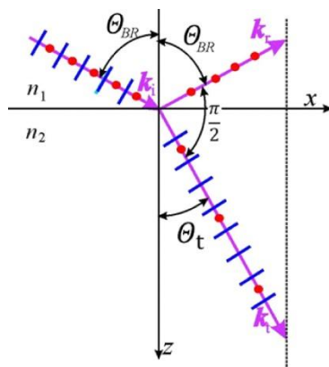
Obr. 2.9 Schématické znázornění principu polarizace odrazem na rozhraní dvou prostředí
