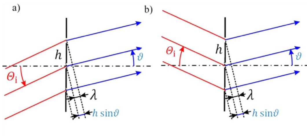
Obr. 6.27 Šikmý dopad rovinné vlny na mřížku. V případě a) jsou úhel dopadu \theta_i i difrakční úhel \vartheta kladné. V případě b) je úhel \theta_i záporný.
