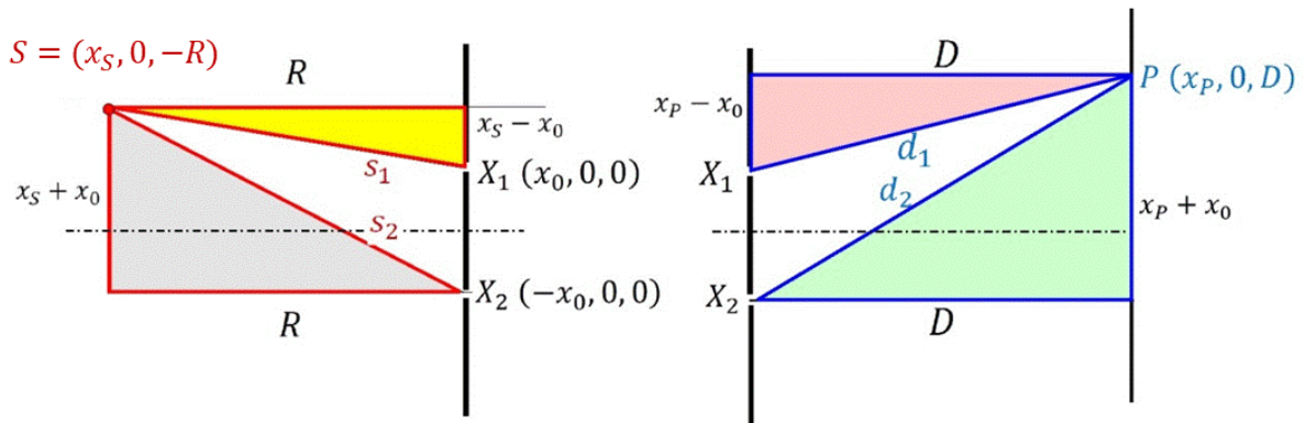
Obr. 7.6 Pravoúhlé trojúhelníky k určení s_2 - s_1 a d_2 - d_1
