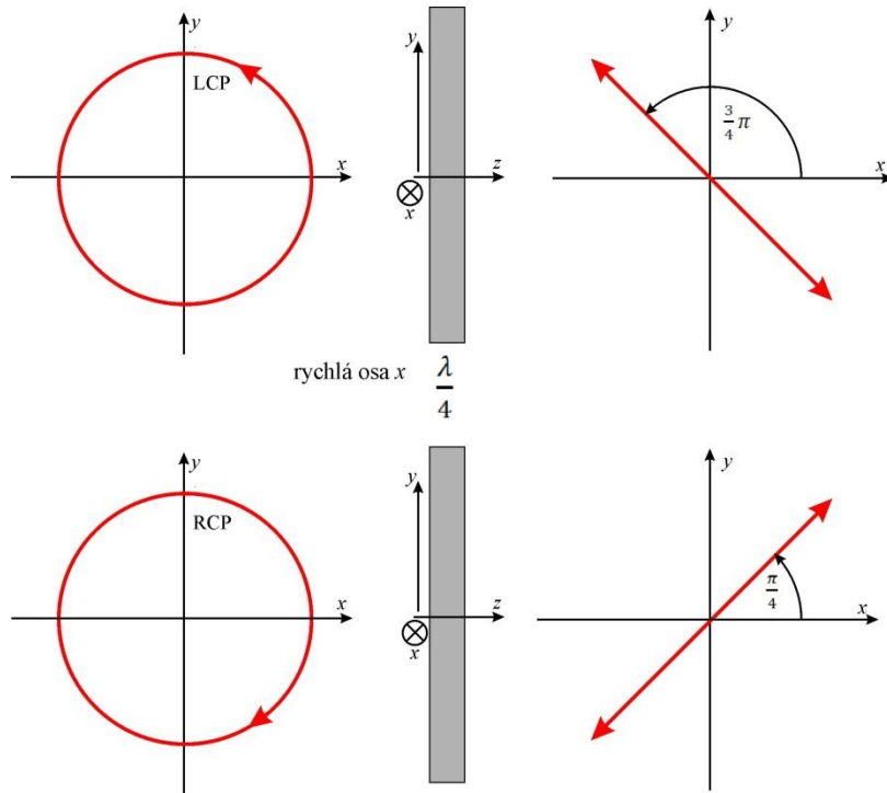
Obr. 2.14 Schématické znázornění působení čtvrtvlnové destičky na kruhově polarizovanou vlnu.
