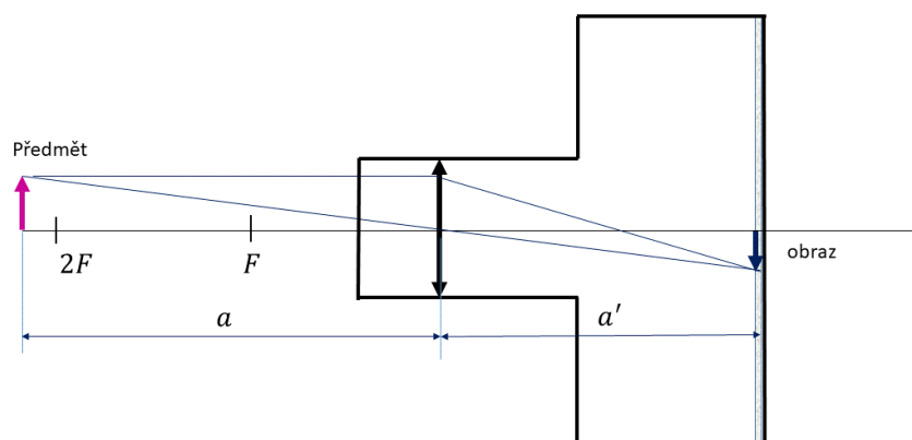
Obr. 8.40 Fotoparát – jednoduché schéma zobrazení předmětu na detektor (fotocitlivý film, matice CCD detektorů)
