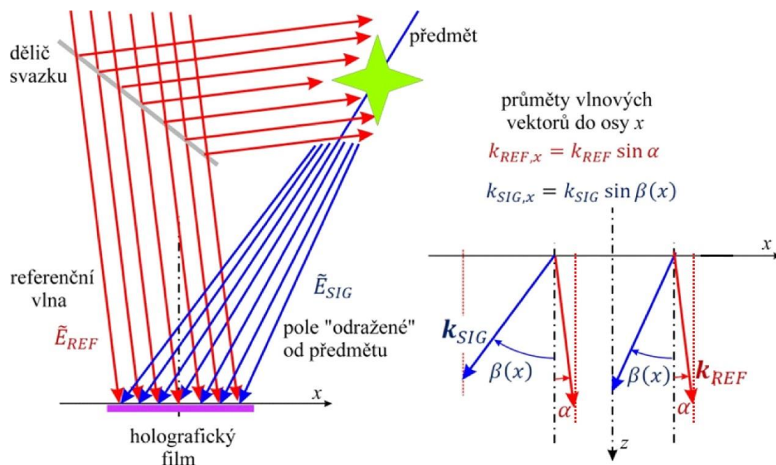
Obr. 6.31 Schéma pro holografický záznam a vlnové vektory referenční vlny a signálních vln
