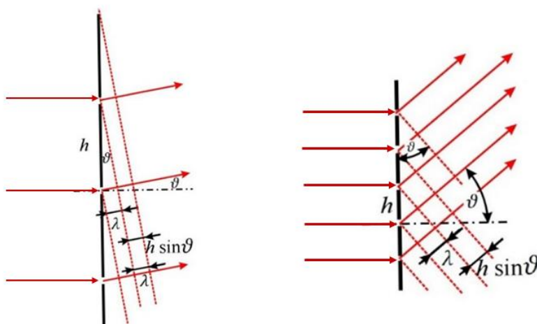
Obr 6.26 Souvislost mezi úhlem \vartheta_{MAX 1} a vzdáleností štěrbin. Pro velká h je dosaženo podmínky maxima h \sin \vartheta_{MAX 1} = \lambda pro m = 1 při menších úhlech \vartheta než pro malá h .
