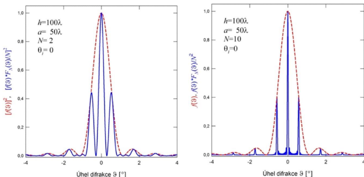
Obr. 6.28. Modelový průběh intenzity světla po difrakci na difrakční mřížce v závislosti na počtu štěrbin N = 2 a 10 a pro šířku štěrbin a = \frac{h}{2} . Červená přerušovaná křivka reprezentuje úhlovou závislost difrakční intenzity (s difrakčními maximy) pro 1 štěrbinu f_1^2(\vartheta) = \left(\frac{\sin u}{u}\right)^2 která představuje obálku pro interferenci souboru identických štěrbin \sim F_N^2 (s interferenčními maximy). Intenzita ve výsledném obrazci je úměrná součinu obou funkcí.
