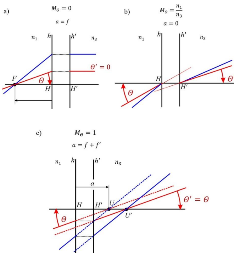
Obr. 8.27 Příklady úhlového zvětšení. a) Předmětová přímka prochází předmětovým ohniskem M_\theta = 0 . b) Předmětová přímka prochází hlavním bodem M_\theta = \frac{n_1}{n_3} . c) Předmětová přímka prochází uzlovým bodem M_\theta = 1 .
