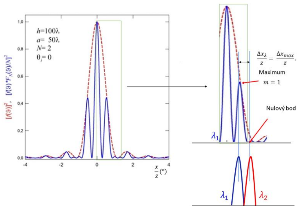
Obr. 6.37 Spektrální rozlišení difrakční mřížky demonstrované pro případ 1. maxima ( m=1 ). Dvě světelné vlny s vlnovými délkami \lambda_1 a \lambda_2 procházející difrakční mřížkou jsou na detektoru umístěném ve vzdálenosti z rozlišitelné, pokud jsou jejich 1. maxima vzdálená ( \Delta x_\lambda ) o pološířku maxima pro \lambda_1 (vzdálenost mezi maximem a 1. nulovým bodem), \Delta x_\lambda = \Delta x_{max} .
