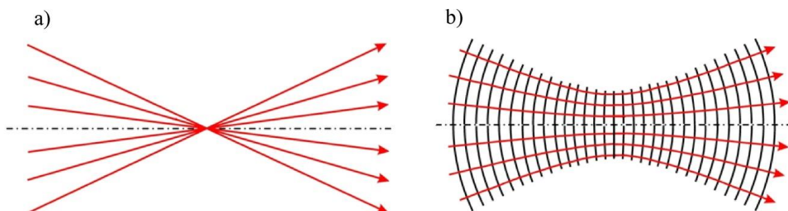
Obr. P8.4.1 a) Znáznornění fokusace rovnoběžného svazku v modelu paprskové optiky. b) Rozložení intenzity v ohniskové rovině ve skalárním modelu Fraunhoferovy difrakce, viz též obr. 6.18.
