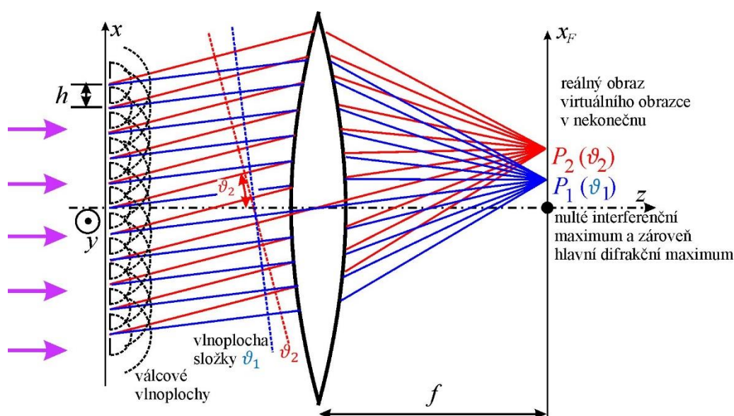
Obr. 6.25 Virtuální interferenční obrazec N rovinných vln v nekonečnu je složen z rovinných komponent charakterizovaných úhlem \vartheta . Tento obrazec si můžeme „přitáhnout“ do ohniskové roviny fokusační optiky. Předpokládáme, že na mřížku dopadá rovinná vlna s vlnovým vektorem rovnoběžným s osou z (úhel dopadu \theta_i = 0 ), takže pole ve všech štěrbinách kmitají ve fázi. Intenzita v ohniskové rovině je určena úhlem \vartheta . Nulté interferenční maximum je na ose z , x_F = 0 pro všechny vlnové délky. Je možná např. situace, že pro některou vlnovou délku je v P_1 interferenční minimum a v P_2 první hlavní interferenční maximum.
