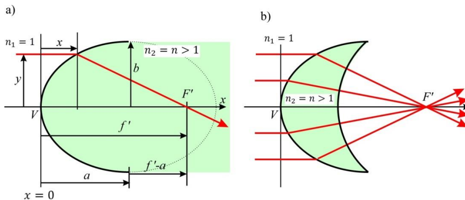
Obr. P8.5.1 Fokusace rovnoběžného svazku lomnou plochou elipsoidu. a) Základní geometrické uspořádání. b) Praktické provedení ve tvaru aplanatického menisku, kdy na druhé ploše (kulové se středem v F' ) nedochází k lomu.
