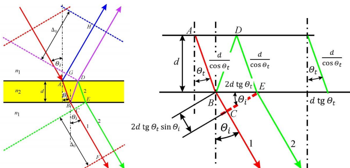
Obr. P.4.1.1 Paprskový model dvojsvazkové interference rovinné vlny na planoparalelní dielektrické desce. Vpravo znázorněny geometrické vzdálenosti pro určení rozdílu optických drah.
