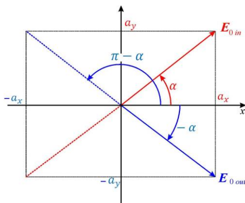
Obr. 2.16 Rotace lineárně polarizovaného světla při průchodu polovlnovou destičkou
