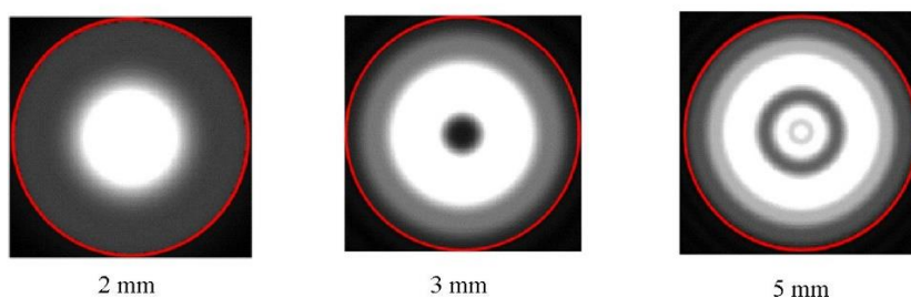
Obr 6.16 Spočtený difrakční obrazec Fresnelovy difrakce na kruhových otvorech uvedených průměrů od 2 mm do 5 mm na matnici vzdálené 4 m od stínítka, vlnová délka světla 515 nm (zobrazeno černobíle). Vně červeného kruhu se nachází oblast geometrického stínu, kde je intenzita oscilací difrakčního obrazce sice nenulová, ale mnohem menší než ve znázorněné oblasti. https://www.falstad.com/diffraction
