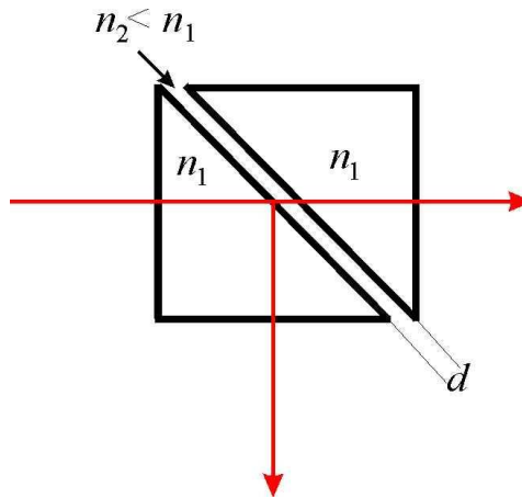
Obr. 3.13 Dvojhranol s mezerou, který může pracovat jako dělič svazku nebo jako regulovatelný vazební člen. Poměr mezi intenzitami vystupujících svazků lze regulovat šířkou šterbiny d .
