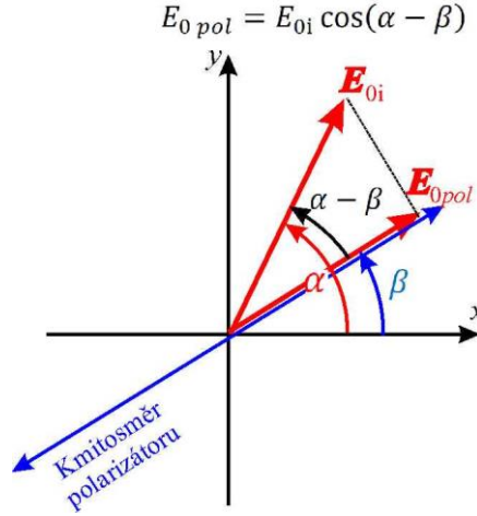
Obr. 2.11 Průchod lineárně polarizovaného světla polarizátorem. E_{0i} je amplituda vlny vstupující do polarizátoru, E_{0pol} je amplituda vlny vystupující z polarizátoru.
