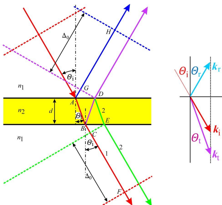
Obr. 4.9 Model dvojsvazkové interference rovinné vlny na planparalelní dielektrické desce. Vpravo je znázorněn zákon odrazu a lomu na prvním rozhraní. Vlnoplocha procházející bodem A potřebuje na proběhnutí dráhy ABC kratší čas než na proběhnutí dráhy ABDE . Totéž vyjádřeno jinak: vlnoplocha procházející body E a C a vlnoplocha procházející bodem F potřebují na dráhu z bodu A stejný čas.
