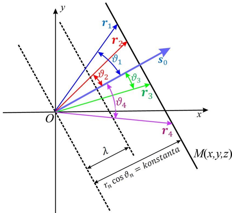
Obr. 1.1 Znázornění řezů rovinných vlnoploch pro vlnu s vlnovým vektorem \mathbf{k} = (k_x, k_y, 0) = k \mathbf{s}_0 . Čárkovaně je zakreslen řez vlnoplochou procházející počátkem souřadné soustavy a řez další vlnoplochou vzdálenou od počátku o vlnovou délku \lambda . Barevně jsou zakresleny čtyři polohové vektory reprezentující obecný polohový vektor bodu na vlnoploše M . Vzdálenosti r_i různých bodů vlnoplochy M od počátku v jednom libovolném čase splňují podmínku \mathbf{s}_0 \cdot \mathbf{r}_i = s_{0x}x_i + s_{0y}y_i = r_i \cos \vartheta_i = vt . Vlnová délka je \lambda = vT , T je doba kmitu.
