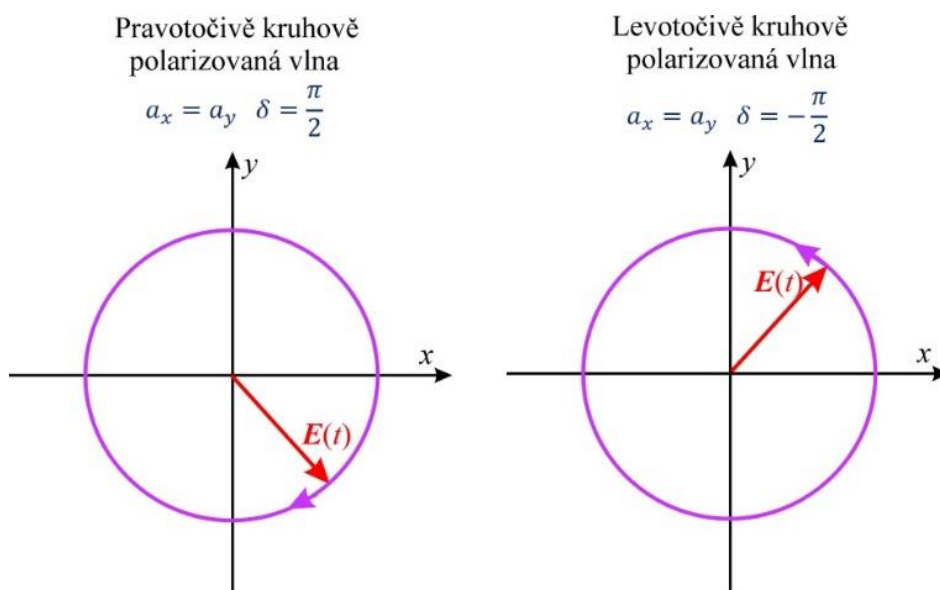
Obr. 2.5 Rotace vektoru elektrického pole v pravotočivě a levotočivě kruhově polarizované vlně v rovině z = konst.
