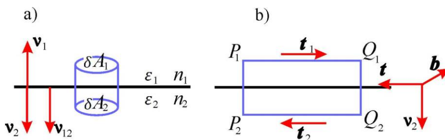
Obr. P.3.1.1 Zavedení veličin pro odvození podmínek na rozhraní
