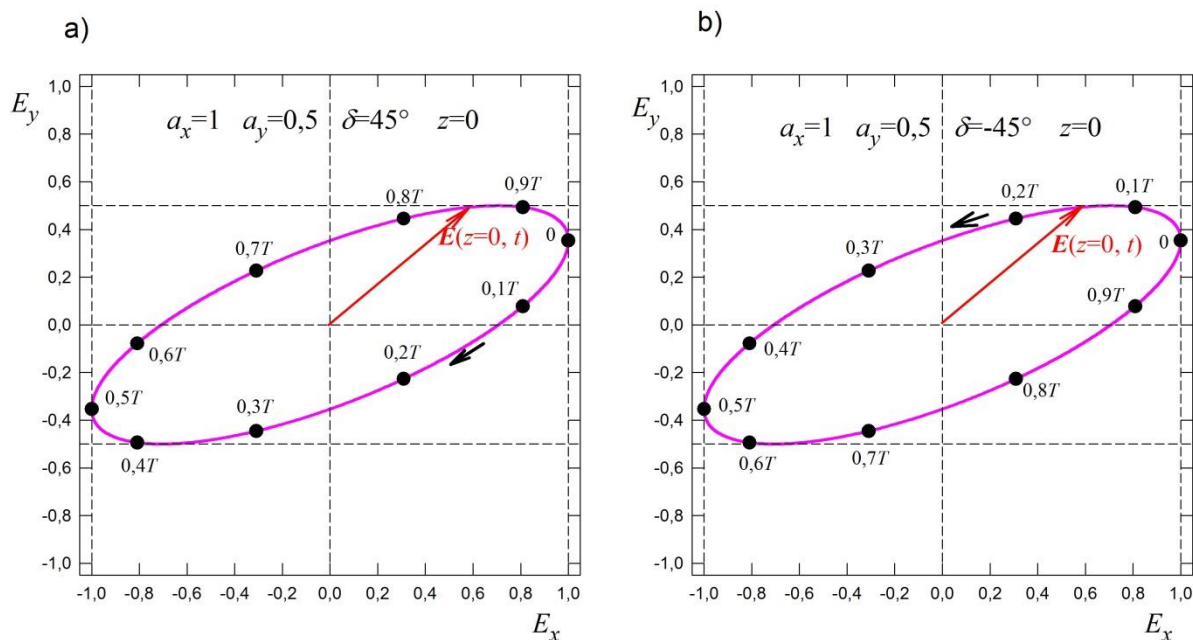
Obr. 2.2 Koncové body vektoru \mathbf{E} se postupně objevují v rovině z = 0 . Znázorněný časový vývoj odpovídá a) vlně pravotočivé, b) levotočivé.
