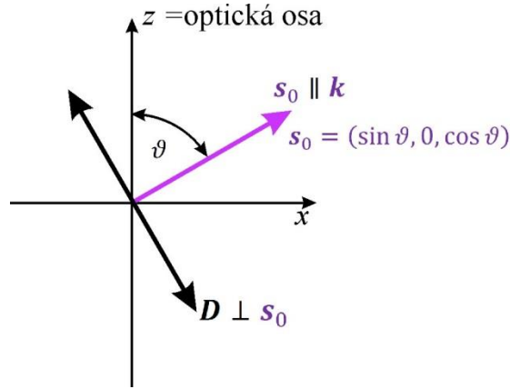
Obr.10.2 Směr vlnového vektoru \mathbf{s}_0 \parallel \mathbf{k} v rovině xz
