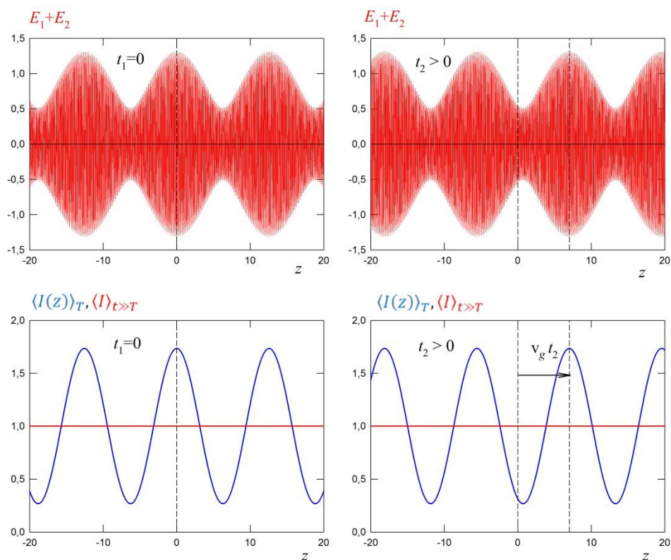
Obr. 5.4 Znázornění posuvu pole složeného ze dvou monochromatických vln různých amplitud. V horním řádku je okamžitá hodnota pole v čase t_1 = 0 a v čase t_2 > 0 . V dolním řádku je modře vyznačena „intenzita“ získaná středováním přes periodu \bar{T} = \frac{2\pi}{\omega} a červeně intenzita zprůměrovaná přes delší časový interval t \gg \bar{T} jako prostorově nezávislá veličina. Možná změna tvaru obálky při šíření v disperzním prostředí není zahrnuta.
