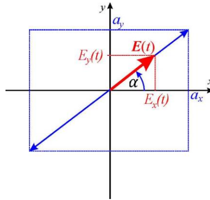
Obr. 2.7 Vektor \mathbf{E} lineárně polarizované vlny a jeho složky
