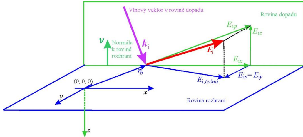
Obr. 3.1 Průběh vektoru elektrického pole (červeně) do roviny rozhraní a do roviny dopadu. Modře jsou zakresleny složky ležící v rovině rozhraní, zeleně v rovině dopadu. Tečná složka k rovině rozhraní \mathbf{E}_{i,tečna} má souřadnice (E_{ix}, E_{iy}, 0) , složka \mathbf{E}_{ip} ležící v rovině dopadu má souřadnice (E_{ix}, 0, E_{iz}) . Pro popis odrazu a lomu je důležité rozložení na komponentu kolmou k rovině dopadu \mathbf{E}_{is} = (0, E_{iy}, 0) a komponentu ležící v rovině dopadu \mathbf{E}_{ip} = (E_{ix}, 0, E_{iz}) .
