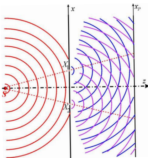
Obr. 7.5 Základní uspořádání interferenčního pokusu podle Younga . Kulové vlny se šíří ze zdroje S a dopadají na malé otvory X_1 a X_2 . Na těchto otvorech dochází k difrakci, tj stávají se zdroji dalších kulových vln, jejichž amplitudy i fáze závisí na amplitudě a fázi dopadající vlny. Čárkovaně je naznačeno přímočaré šíření vlny a je zřejmé, že bez difrakce by se paprsky vycházející ze zdroje a procházející otvory X_1 a X_2 neprotnulý a k žádné interferenci by nedošlo.
