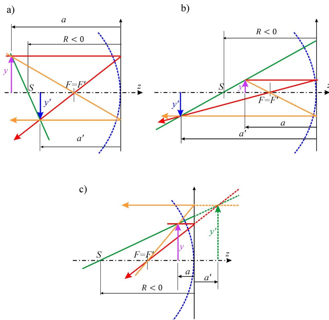
Obr. P.8.7.1 Zobrazení dutým (konkávním) zrcadlem v paraxiální aproximaci
