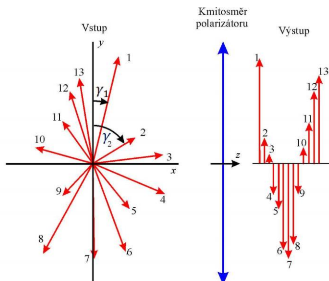
Obr. 2.10 Průchod nepolarizovaného světla polarizátorem. Vektor \mathbf{E} nabývá se stejnou pravděpodobností všech směrů v rovině xy . Úhly \gamma nabývají všech hodnot v intervalu \langle 0, 2\pi \rangle . Na obrázku jsou vyznačeny úhly \gamma_1 a \gamma_2 pro vektory \mathbf{E}_1(t) a \mathbf{E}_2(t) v nějakém časovém okamžiku. V obrázku je naznačen obecnější případ, kdy jednotlivé vlny mají různé amplitudy. Výpočet vedoucí k rovnici (2.18) předpokládá stejnou amplitudu vln E_0 .
