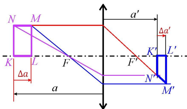
Obr. 8.29 Znáznornění podélného zvětšení pro tenkou spojnou čočku ve vzduchu. Obrazem obdélníka KLMN o podélném rozměru \Delta a je lichoběžník K'L'M'N' podélného rozměru \Delta a' .
